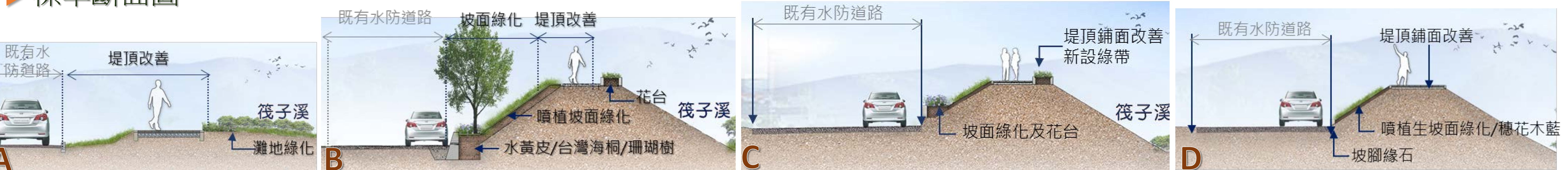
標準斷面圖
