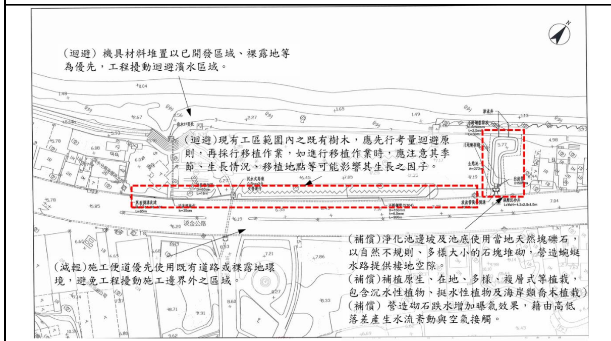
工程平面配置圖
