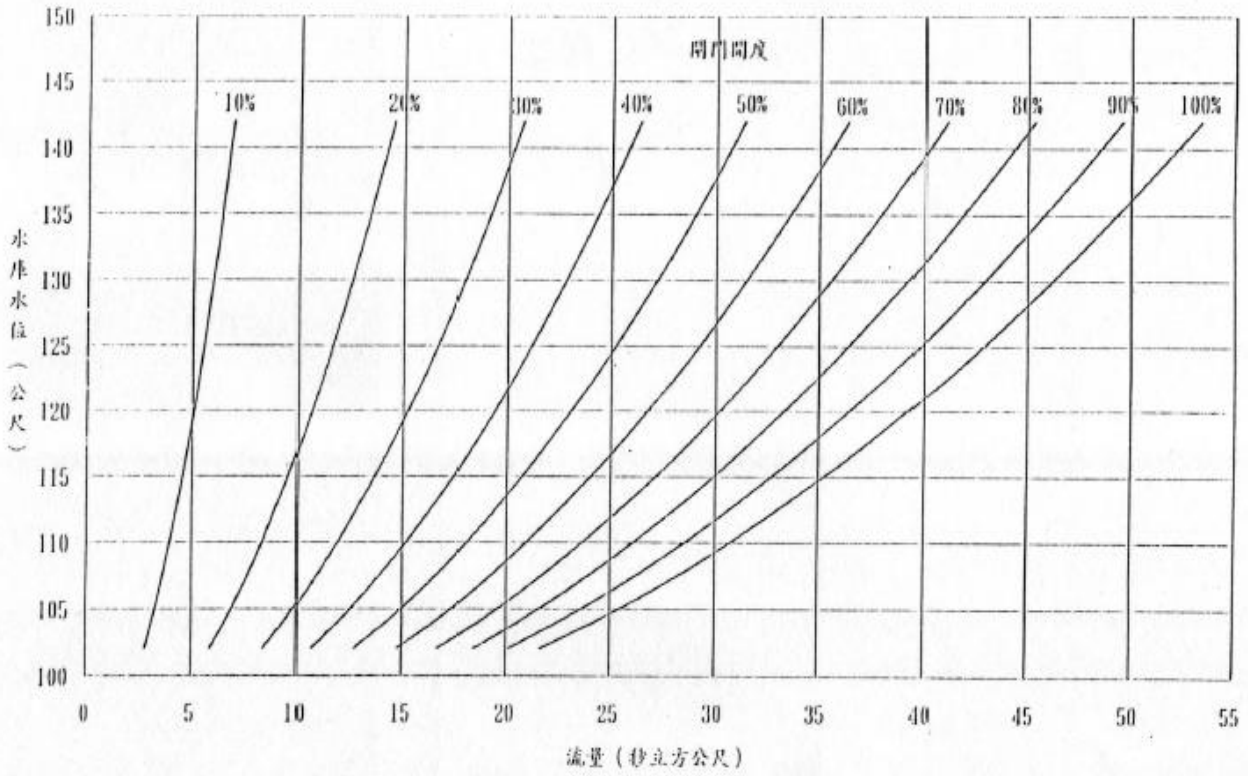
圖三：排水道控制閘門開度與放流量關係曲線
