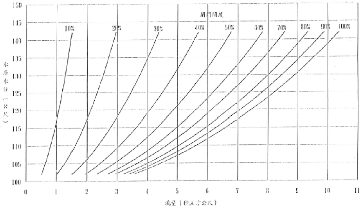
圖四：何本閘開度與放流量關係曲線
