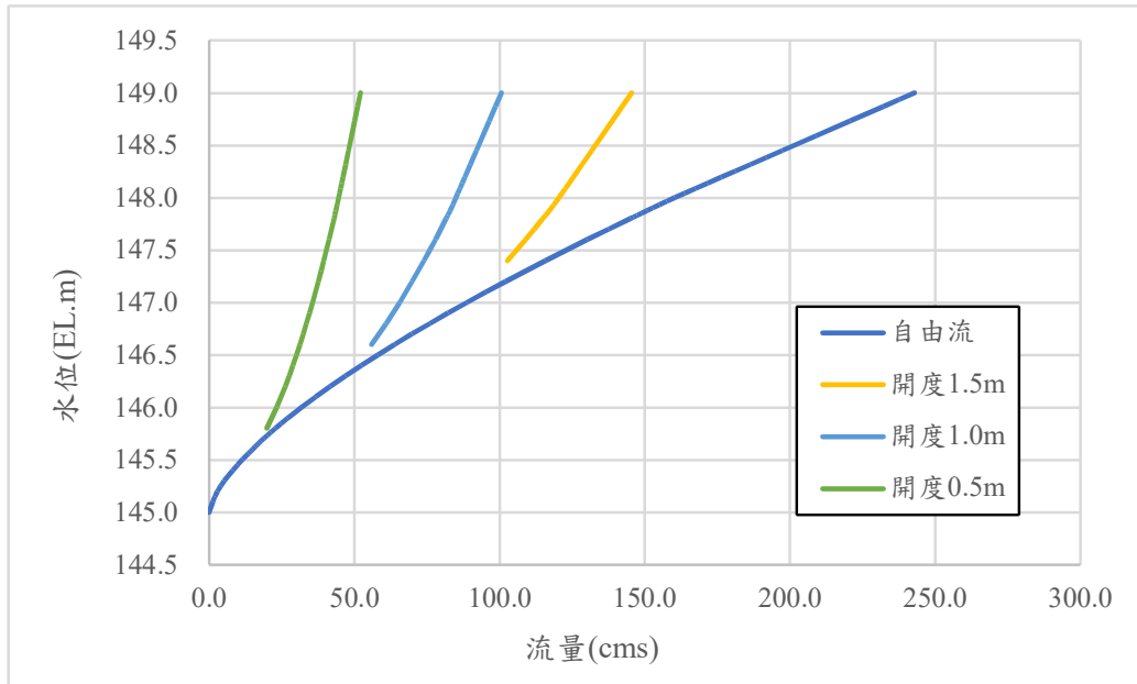
附圖八 取水口開門(開啟三門)水位-開度-流量圖
