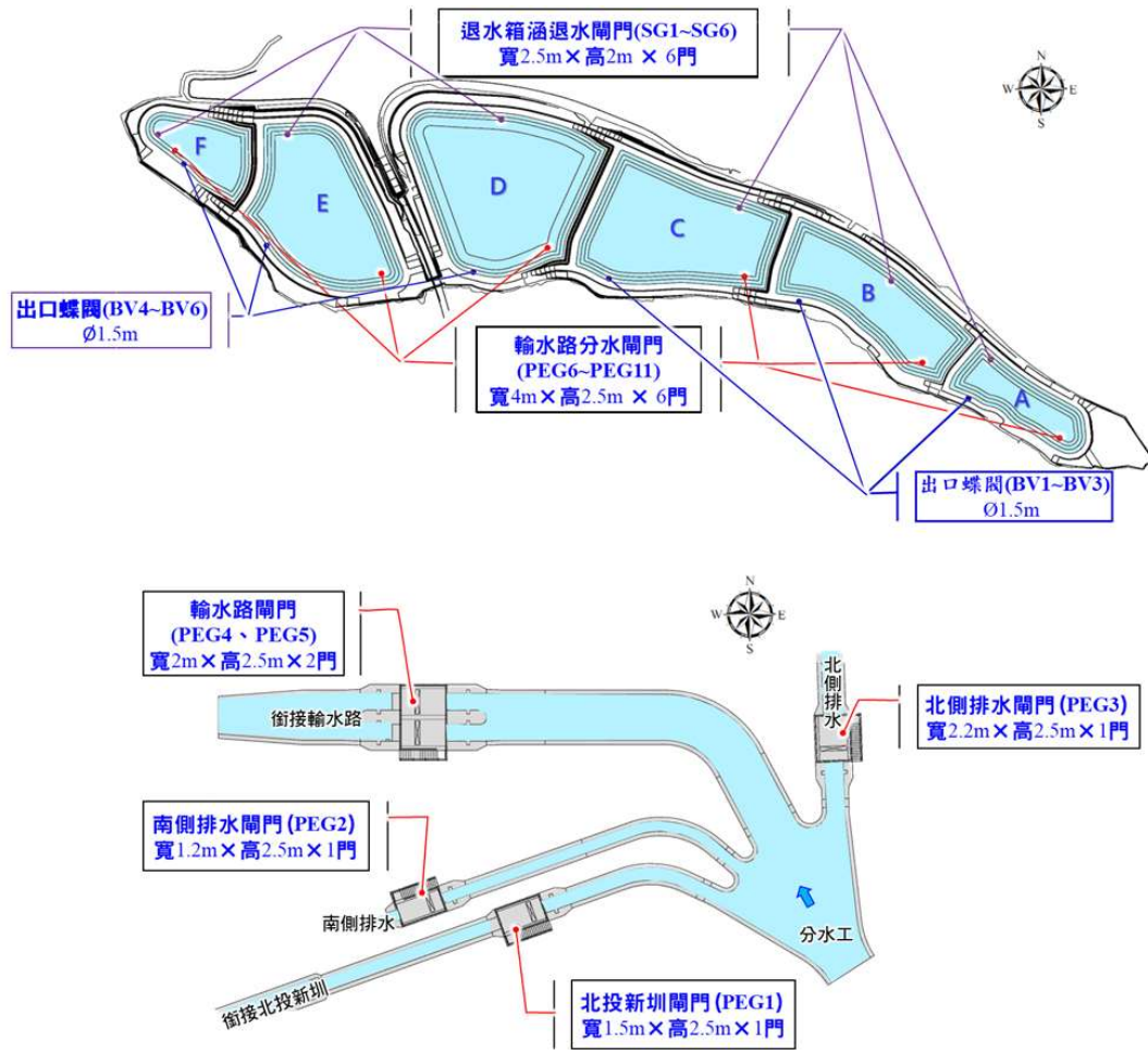
附圖三 人工湖區各設施閘門位置圖
