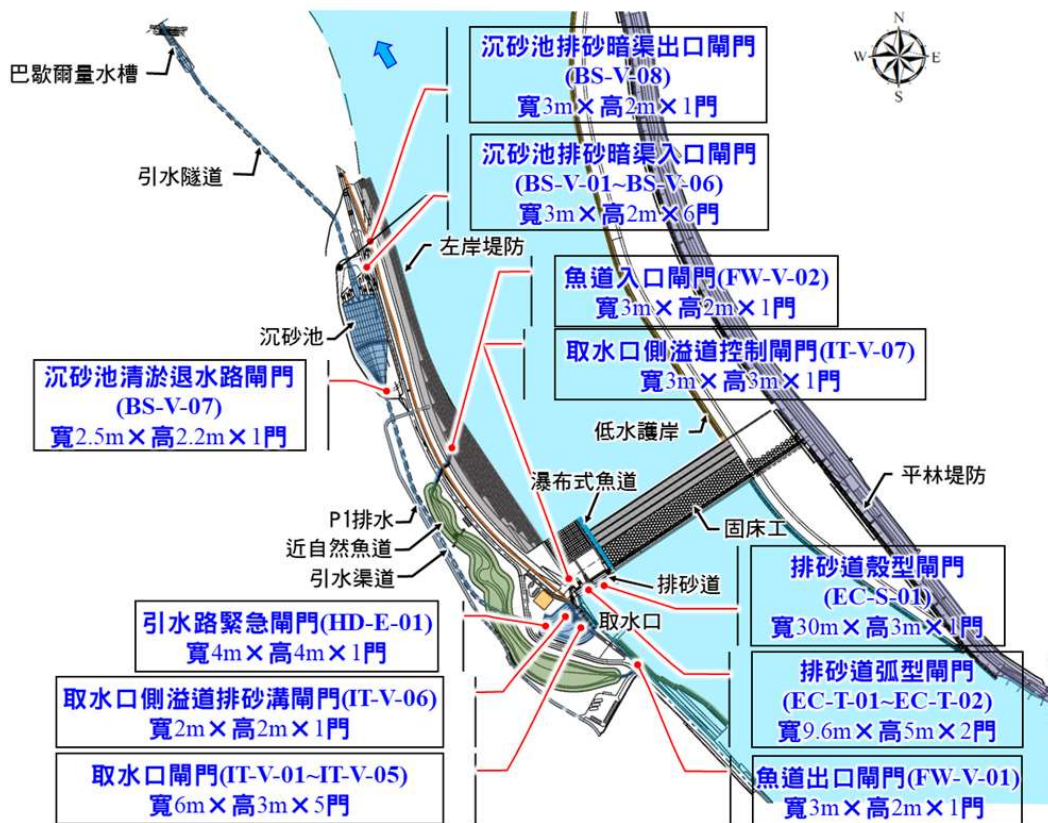
附圖一 烏嘴潭人工湖設施位置圖
