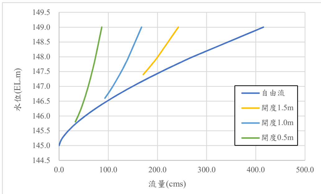
附圖十 取水口開門(開啟五門)水位-開度-流量圖
