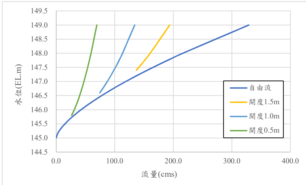
附圖九 取水口開門(開啟四門)水位-開度-流量圖
