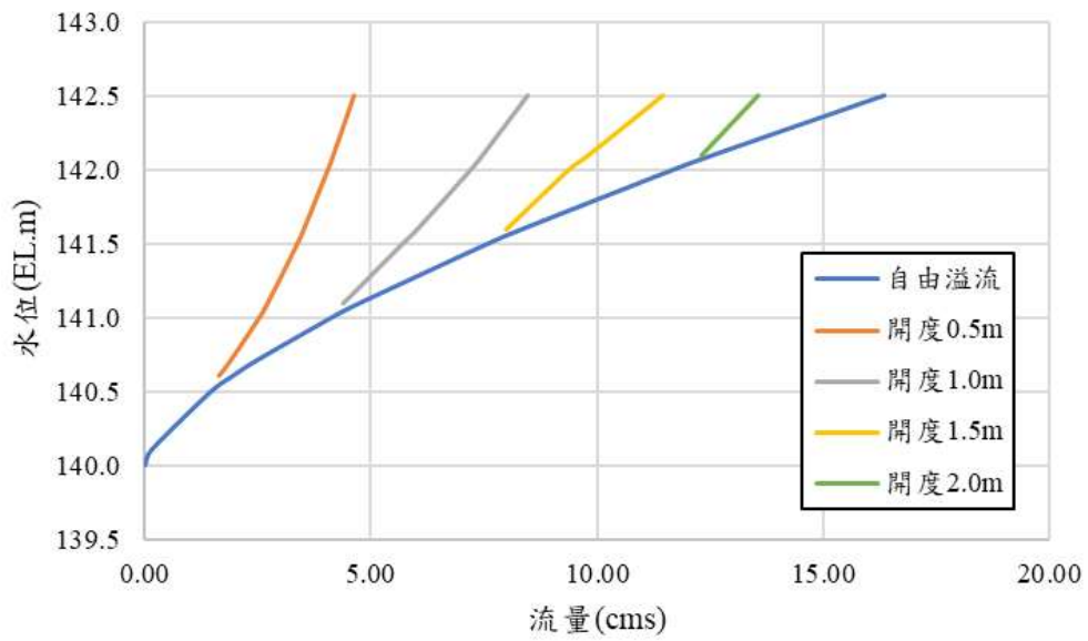
附圖十三 北側排水閘門水位-開度-流量圖
