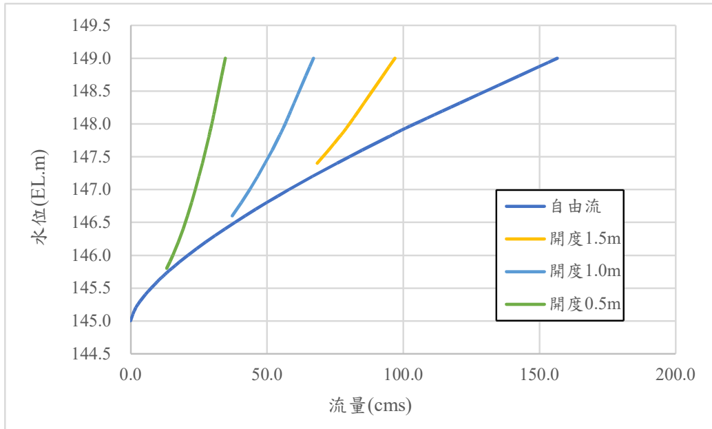
附圖七 取水口開門(開啟二門)水位-開度-流量圖
