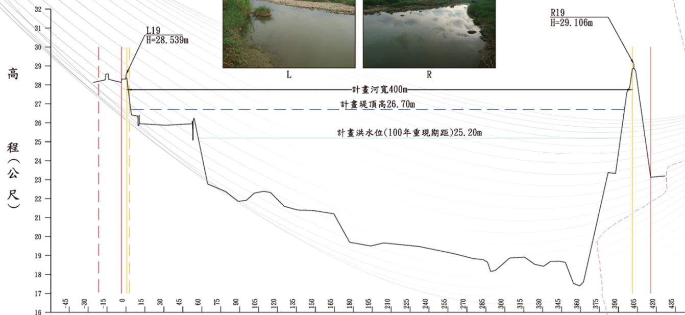
後龍溪橫斷面圖第19號
