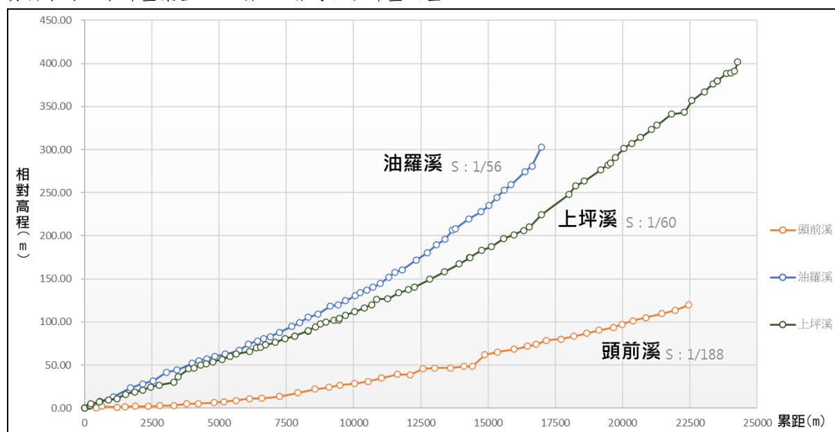
圖 2-6 頭前溪水系河道縱坡示意圖
