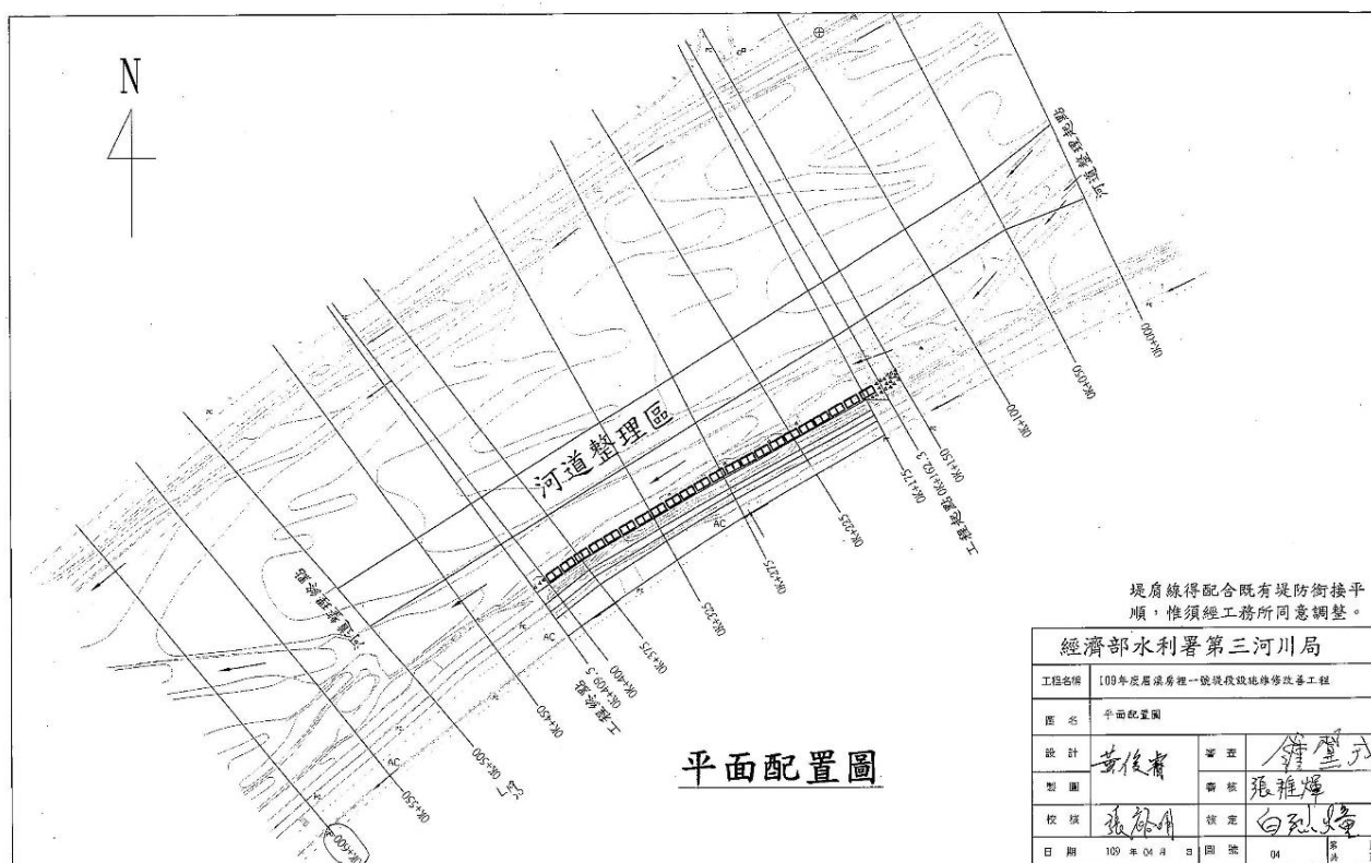
圖 2-1 眉溪房裡一號堤段工區平面圖
