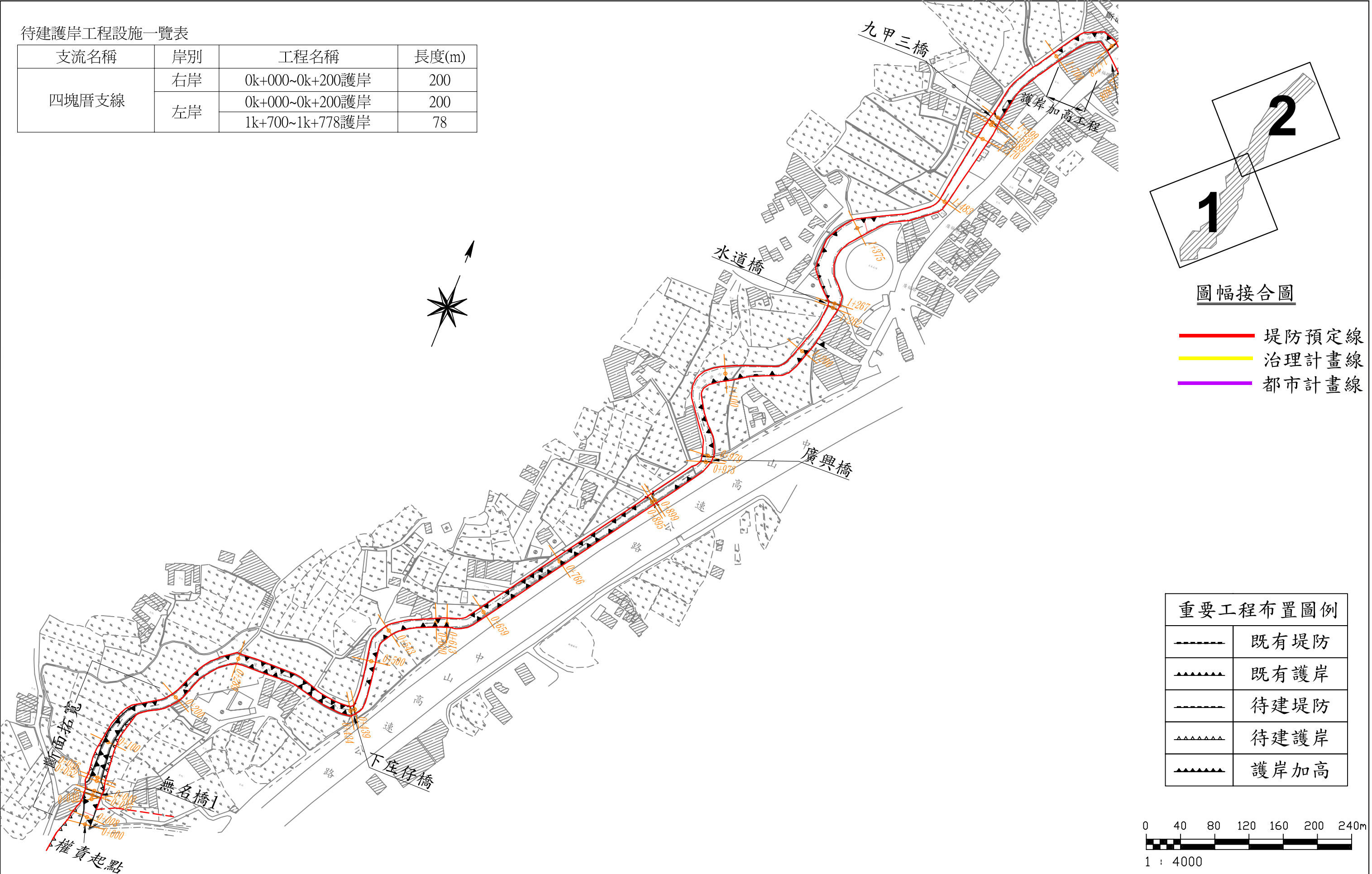
圖14 四塊厝圳支線排水系統工程布置圖(1/2)
