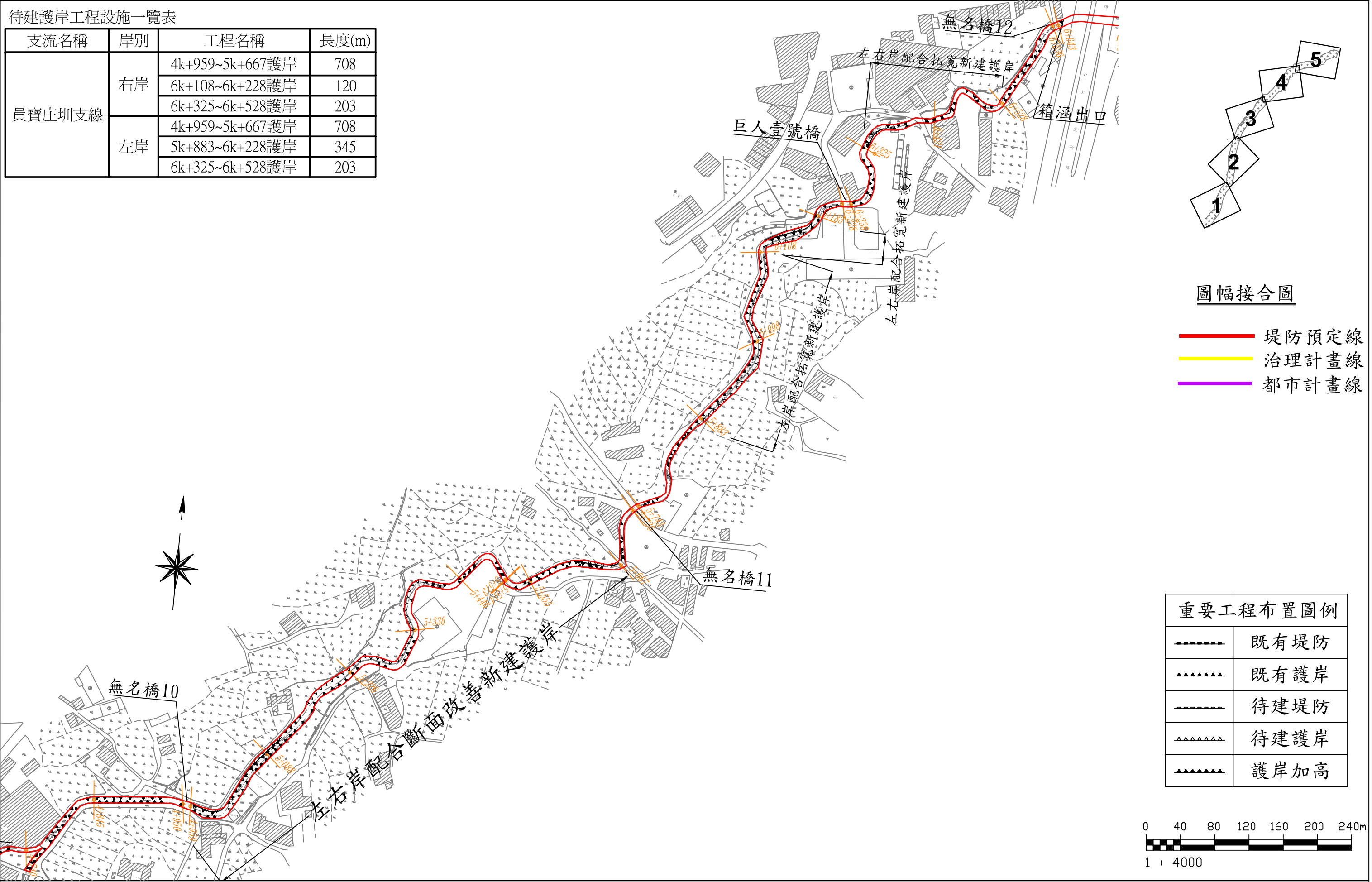
圖16 員寶庄圳支線排水系統工程布置圖(4/5)
