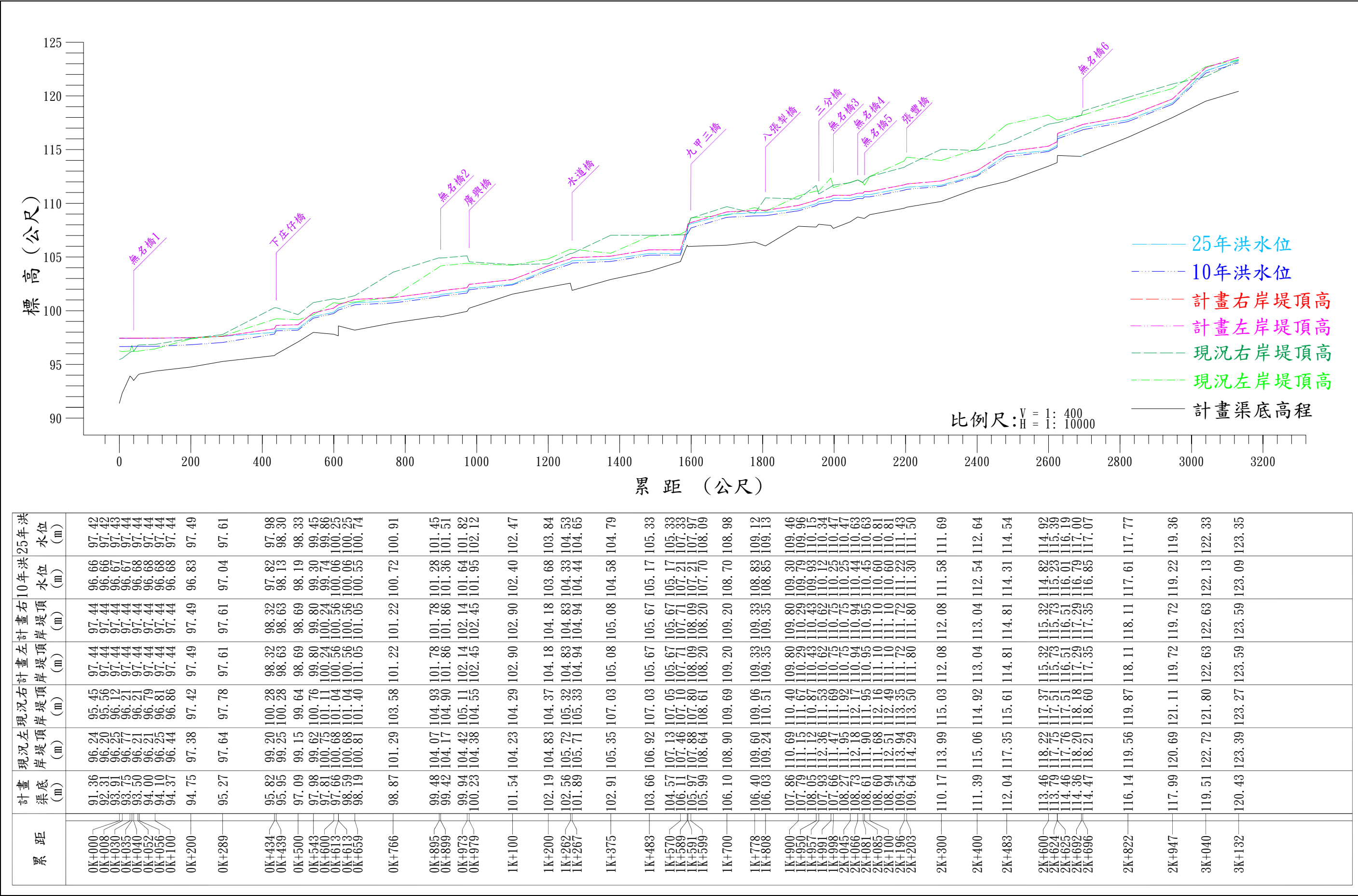
圖4 四塊厝圳支線計畫縱斷面圖
