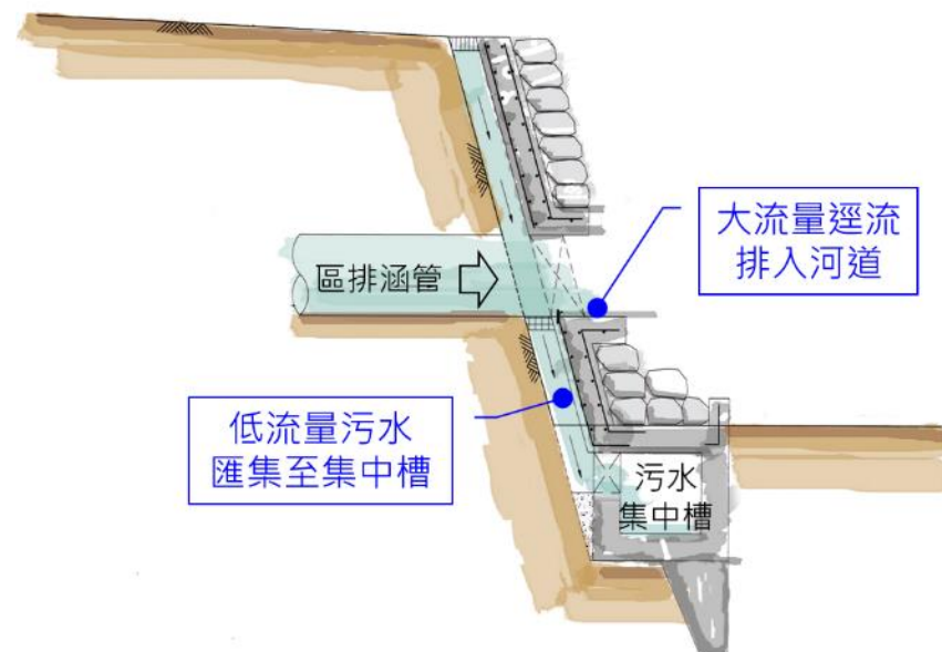
截流設施斷面： • 同聲橋至育英橋
