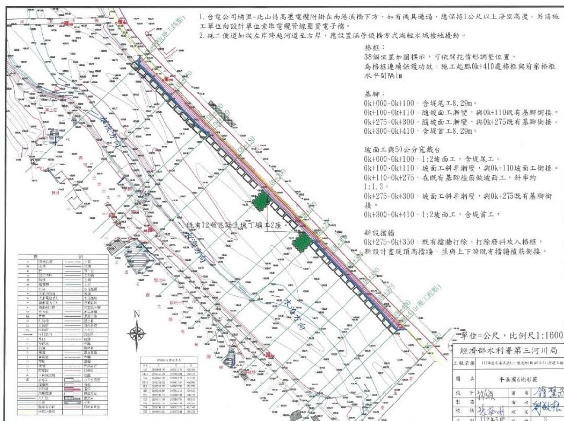
圖3-1 南港溪溪北一號堤防-工程圖
