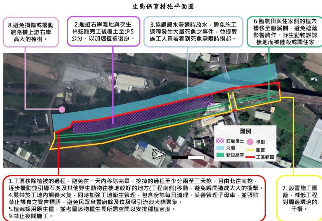
圖3-2 筏子溪農路橋-生態保育措施平面配置圖
