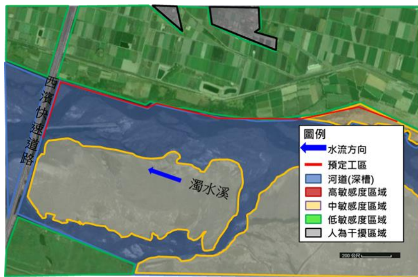
圖 4-129 濁水溪下山腳堤段(斷面 15~21)整建工程生態關注圖
