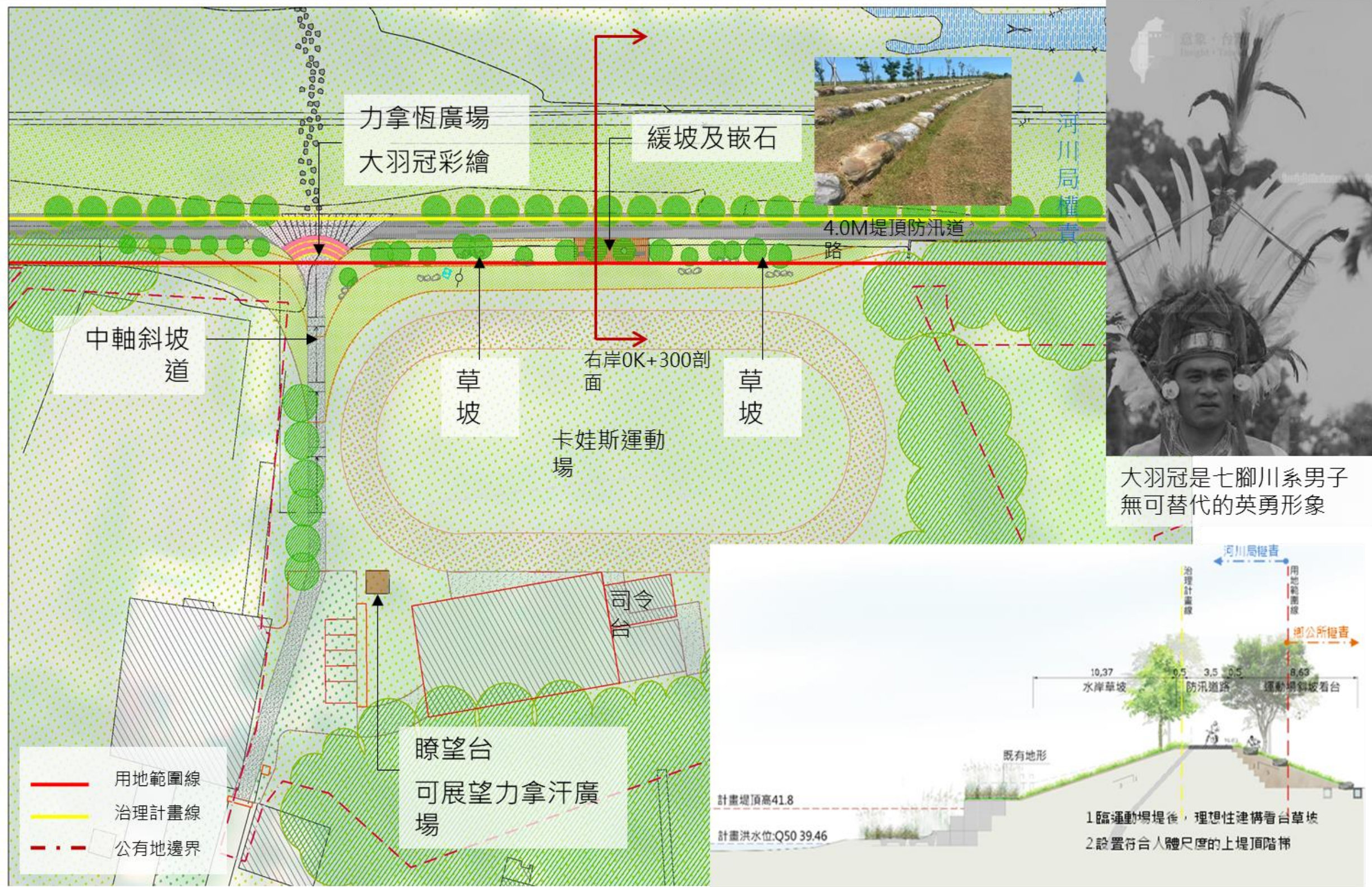
右岸0K+300臨卡娃斯運動場剖面圖(方案一)
