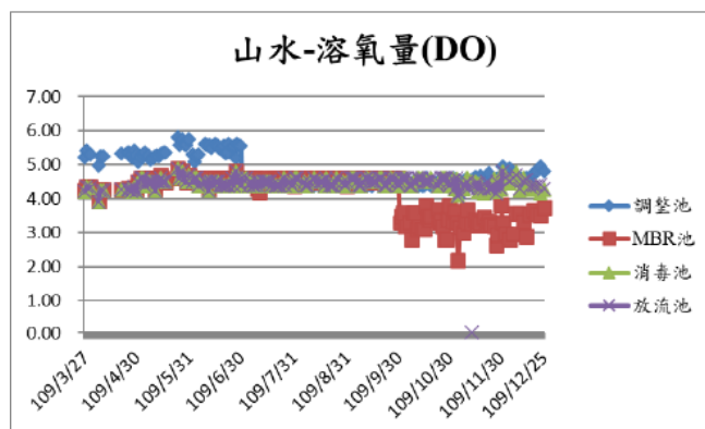
圖附錄 7-2 山水廠各槽池溶氧
