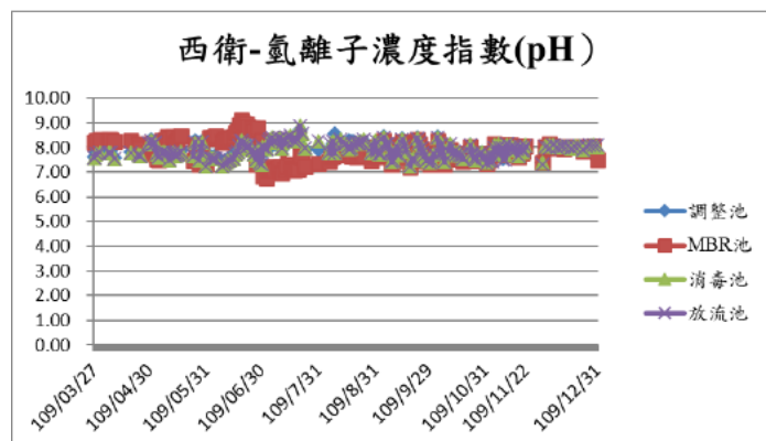
圖附錄 7-5 西衛廠各槽池 PH
