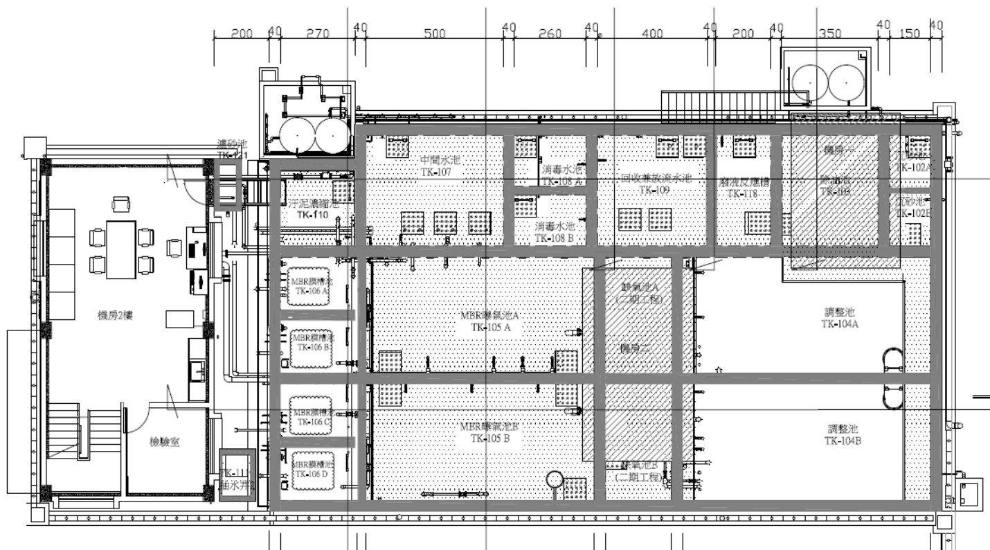
圖 4-7 水資源回收中心配置圖
