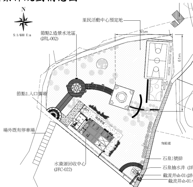
圖 4-5 內灣水質水量調查及水質改善第一期工程配置圖
