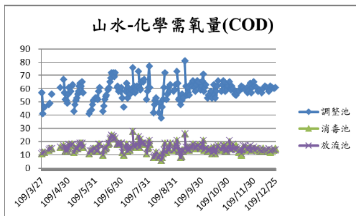
圖附錄 7-4 山水廠各槽池化學需氧量
