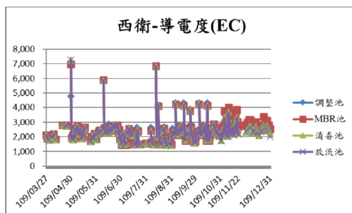
圖附錄 7-3 西衛廠各槽池導電度
