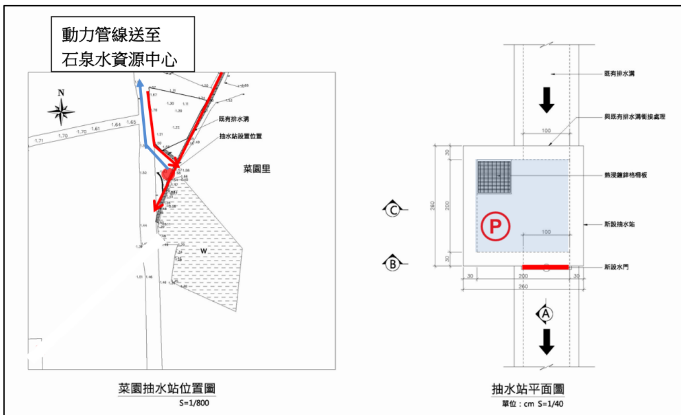
圖 4-11 菜園里截流及抽水站配置圖
