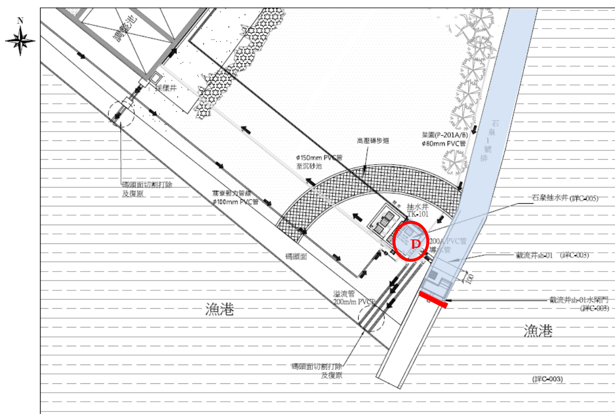
圖 4-12 石泉里截流及抽水站配置圖
