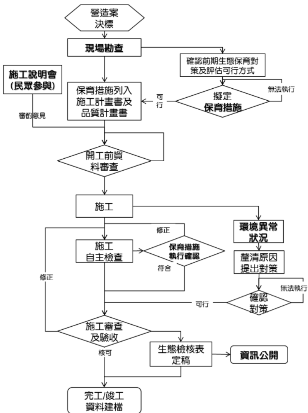
圖 1、施工階段生態評估流程圖
