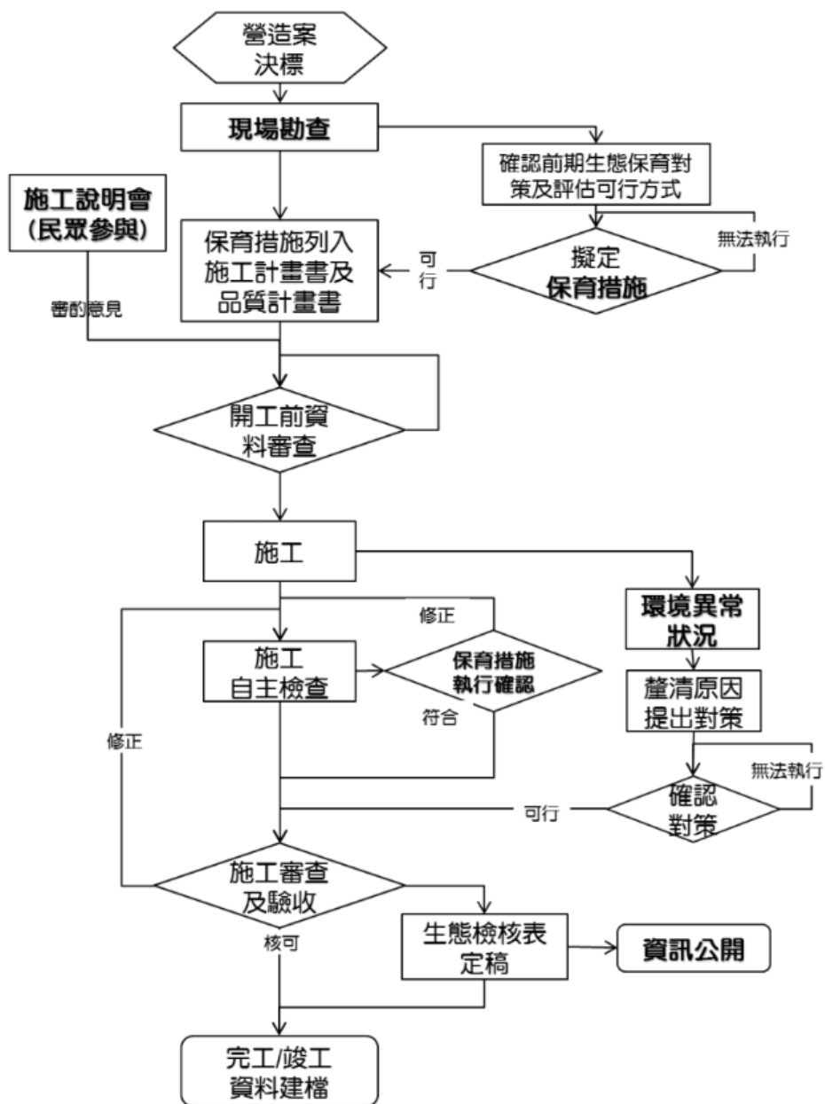
圖 1、施工階段生態評估流程圖
