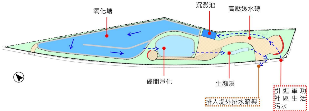
圖 4-2 水質淨化設施工程設計示意圖
