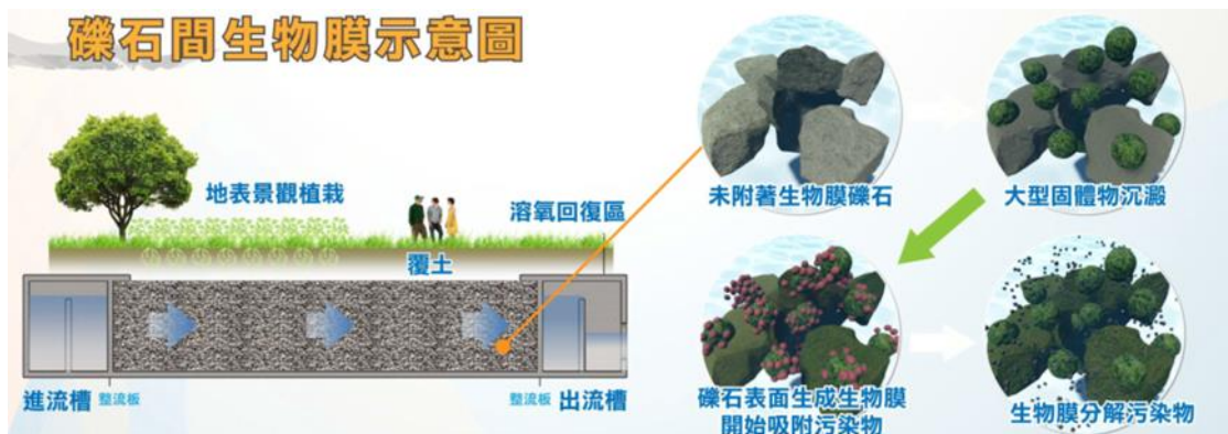
圖 14 礫石間生物處理膜示意圖
