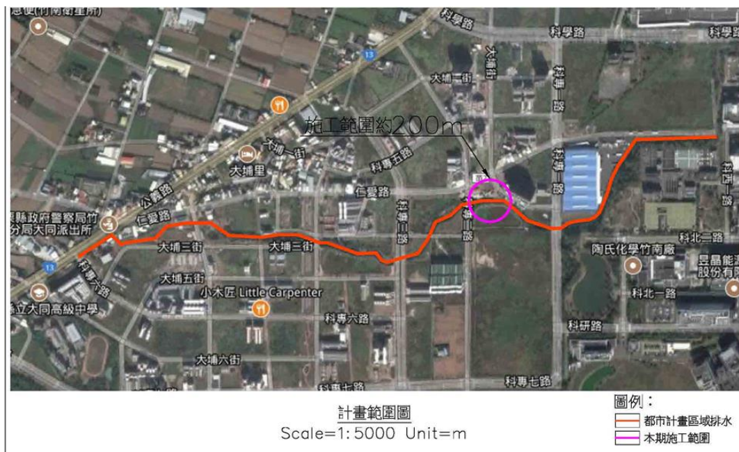
圖 10 滯洪池位置
