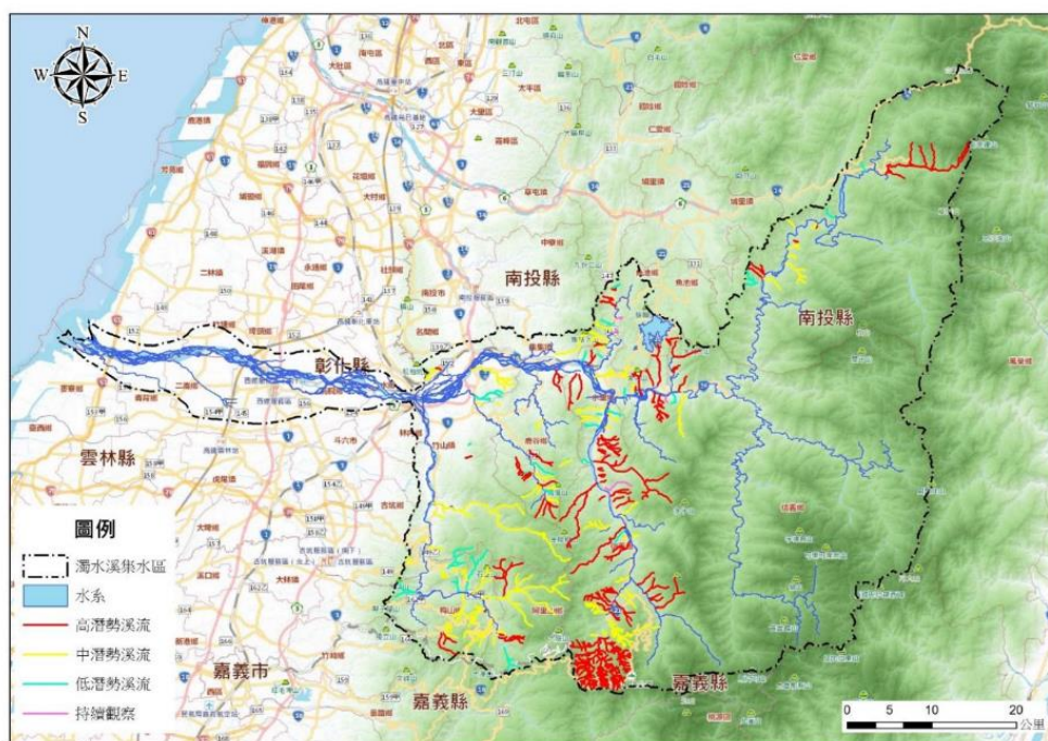
圖 2-16 濁水河流域土石流潛勢溪流分布圖
