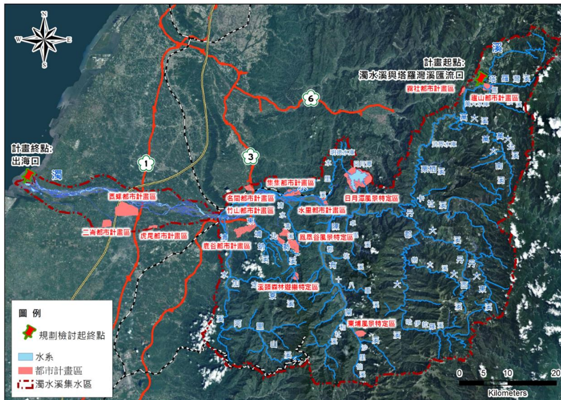
圖 2-38 濁水溪治理規劃河段保全對象分布圖
