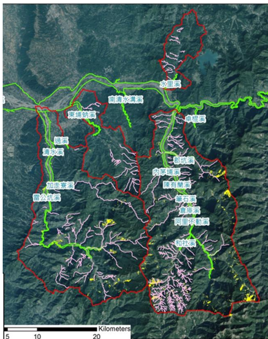
圖 2-36 濁水溪支流流域土石流潛勢溪流與崩塌地位置分布圖
