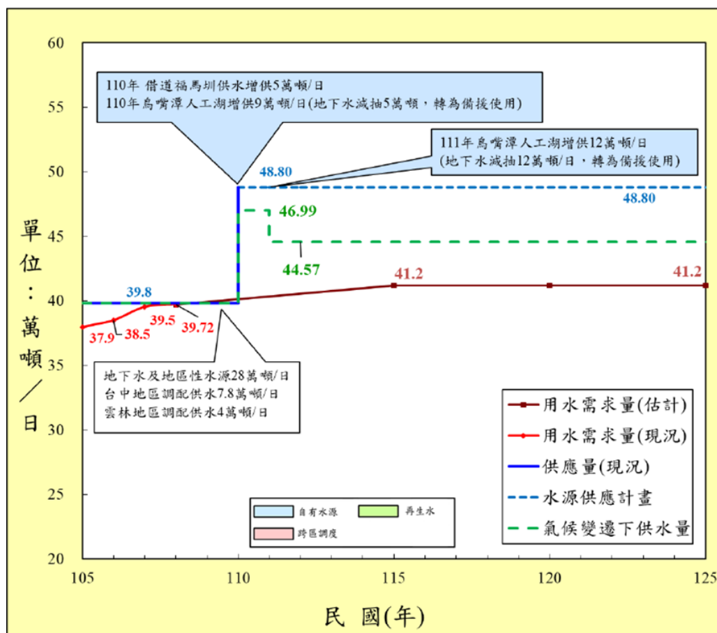
圖 2-23 彰化地區公共給水供需圖
