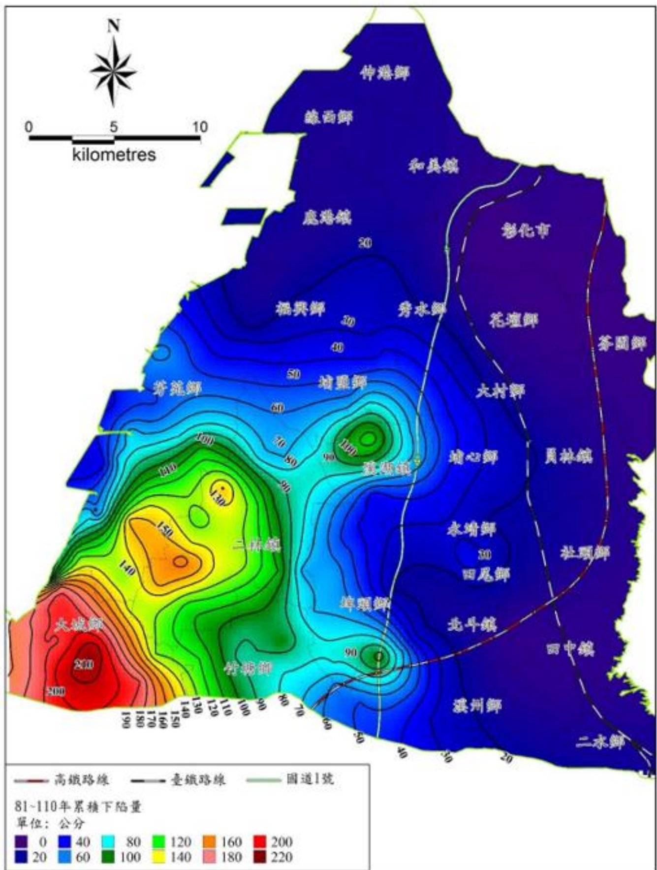
圖 2-53 彰化地區 81~110 年累積下陷量圖
