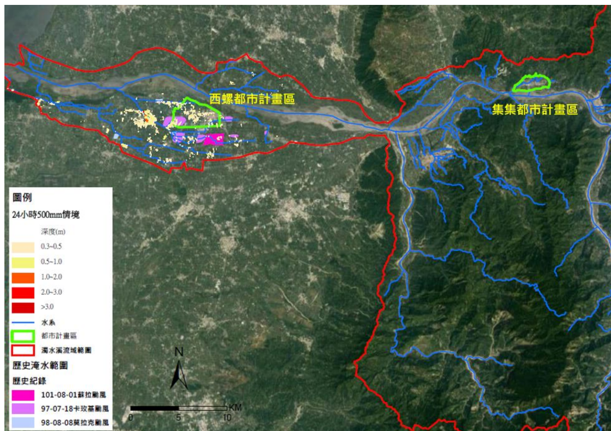
圖 2-48 24 小時 500 毫米情境與歷史淹水紀錄模擬套疊圖
