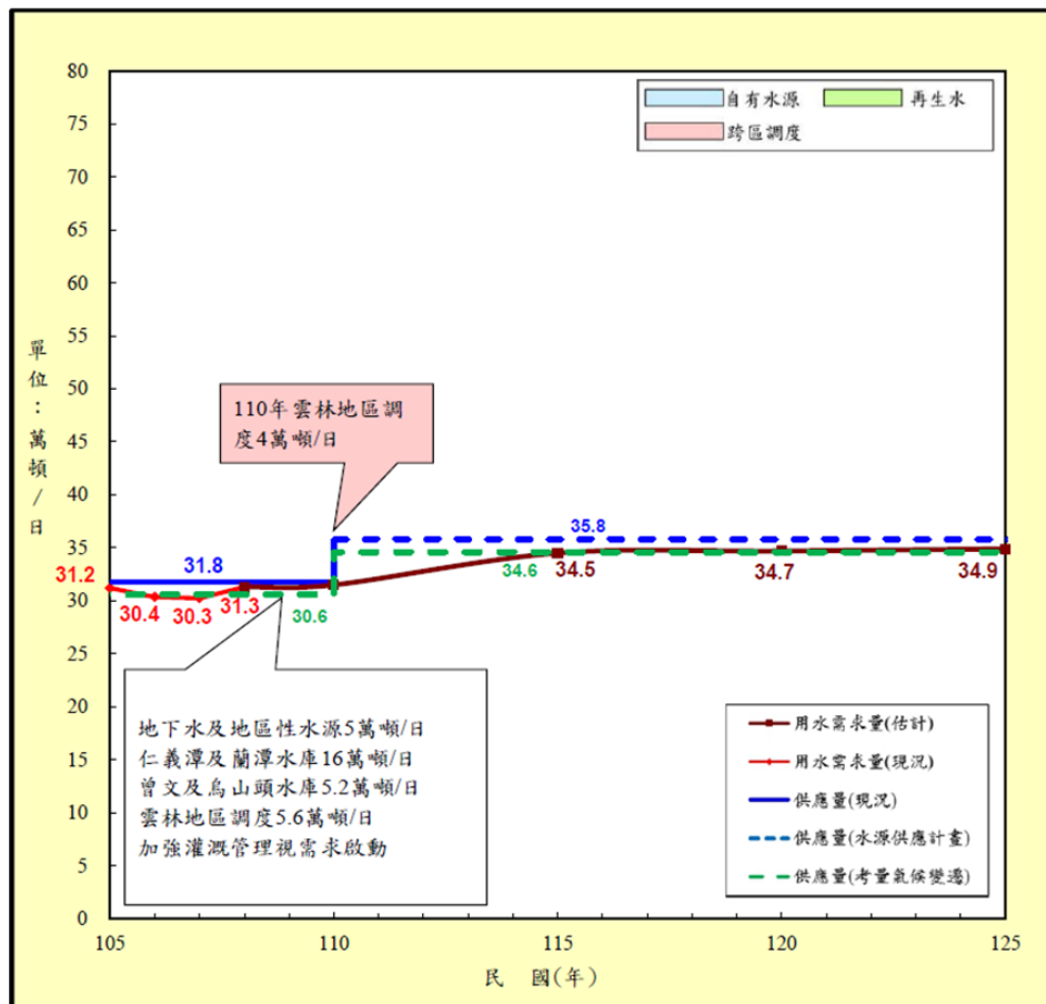
圖 2-25 嘉義地區公共給水供需圖
