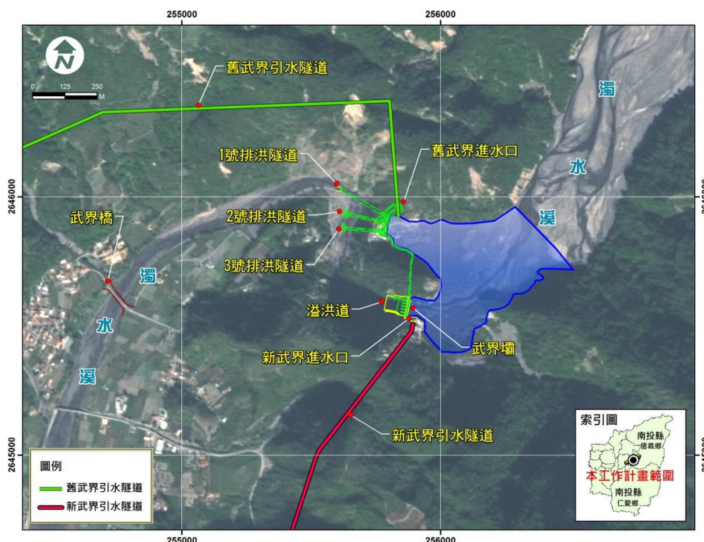
圖 2-30 武界壩水庫右山脊排洪設施現況位置圖
