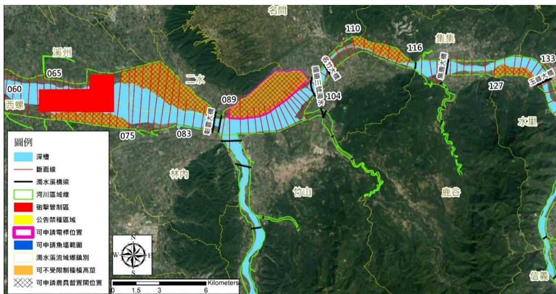
圖 2-47 濁水溪本流許可行為位置分區圖(二)
