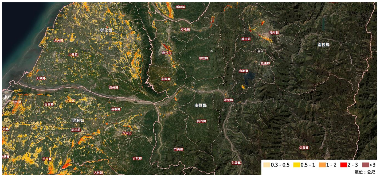
圖 2-39 濁水溪流域 24 小時 500 毫米降雨情境淹水潛勢圖
