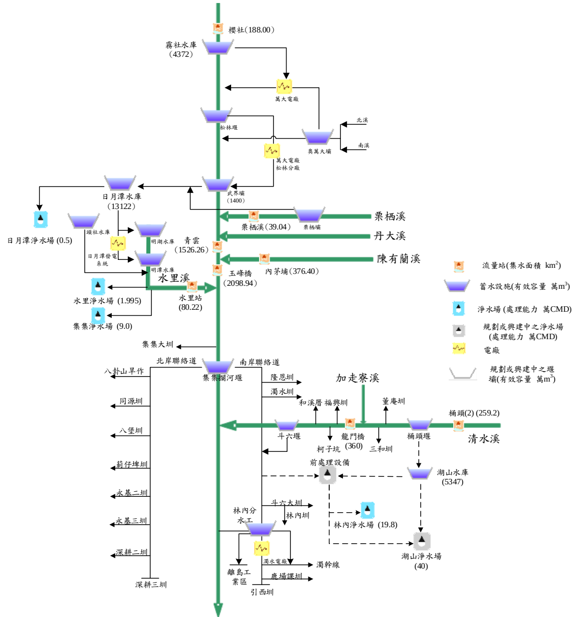
圖 2-28 濁水溪流域水資源設施示意圖
