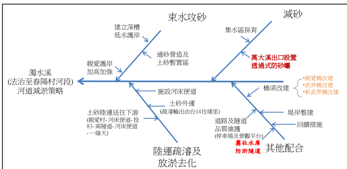
圖 2-77 濁水溪(法治至春陽村)河道減淤策略地圖
