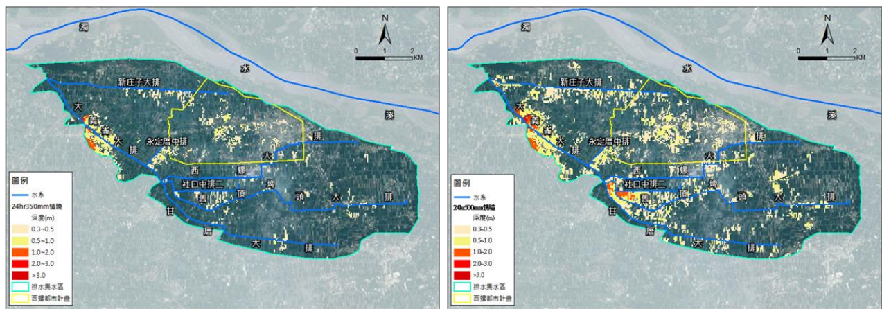
圖 2-42 大義崙排水系統淹水模擬成果
