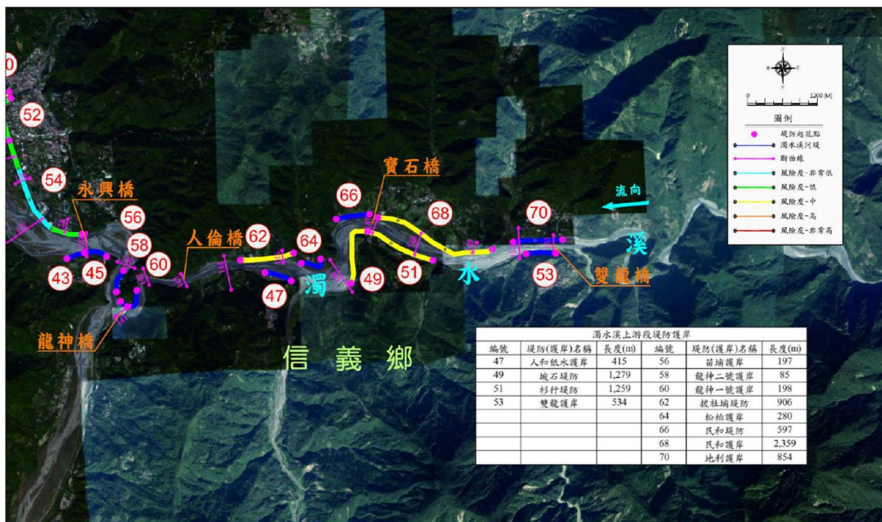
圖 2-34 濁水溪上游段風險度地圖(一)
