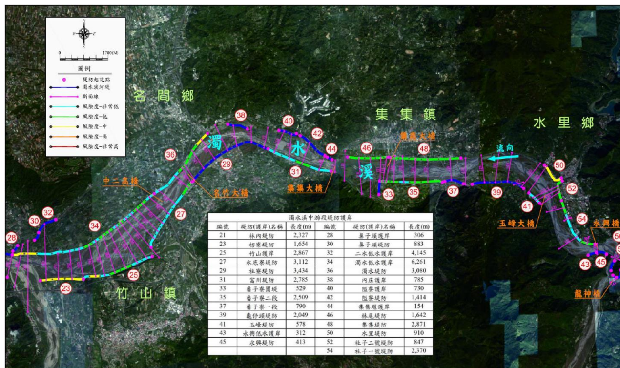
圖 2-32 濁水溪下游段風險度地圖(二)
