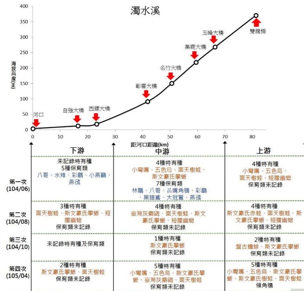
圖 2-59 濁水溪主流陸域生物種類分布圖
