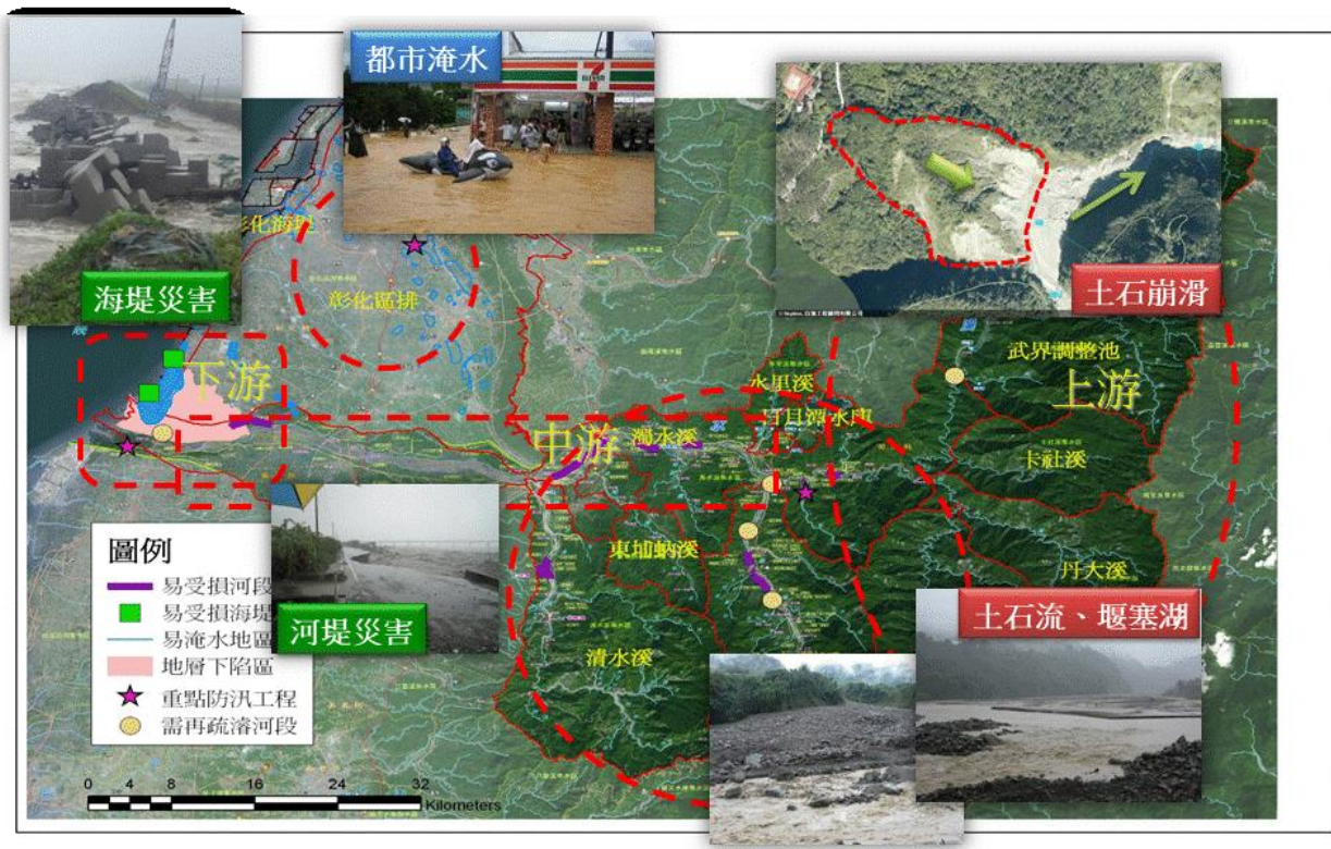
圖 2-29 濁水溪流域災害特性分布圖
