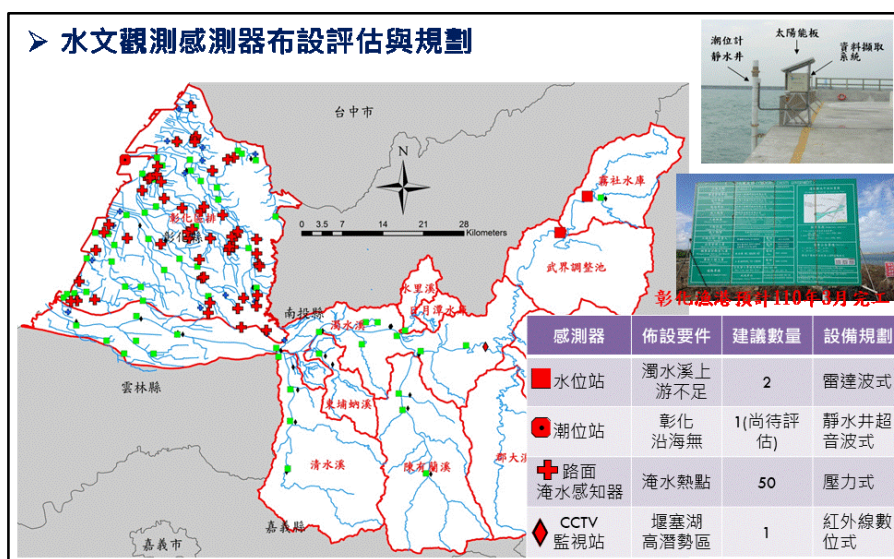
圖 2-51 經濟部水利署第四河川局水文感測器增設建議示意圖
