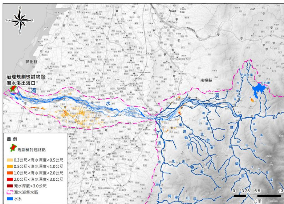
圖 2-12 濁水溪流域 12 小時下降 400 毫米降雨狀況淹水潛勢圖
