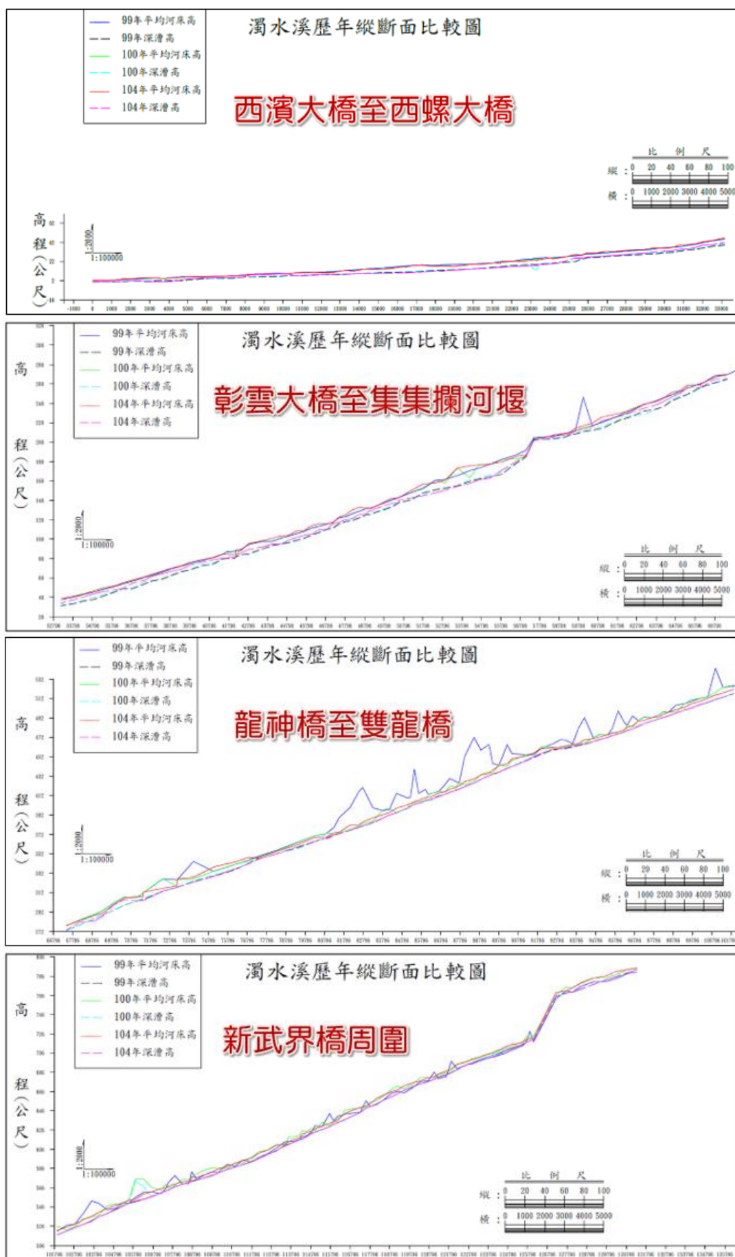
圖 2-7 濁水溪歷年縱斷面高程變化圖
