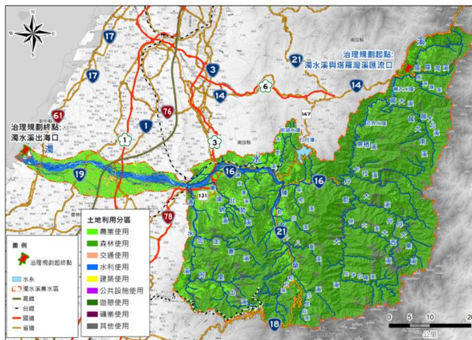
圖 2-10 計畫流域土地利用現況圖
