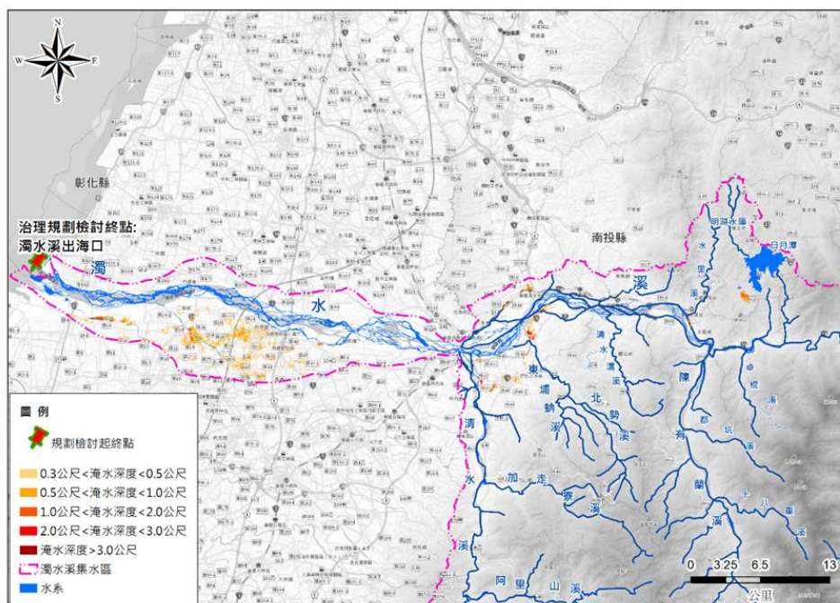
圖 2-11 濁水溪流域 6 小時下降 350 毫米降雨狀況淹水潛勢圖
