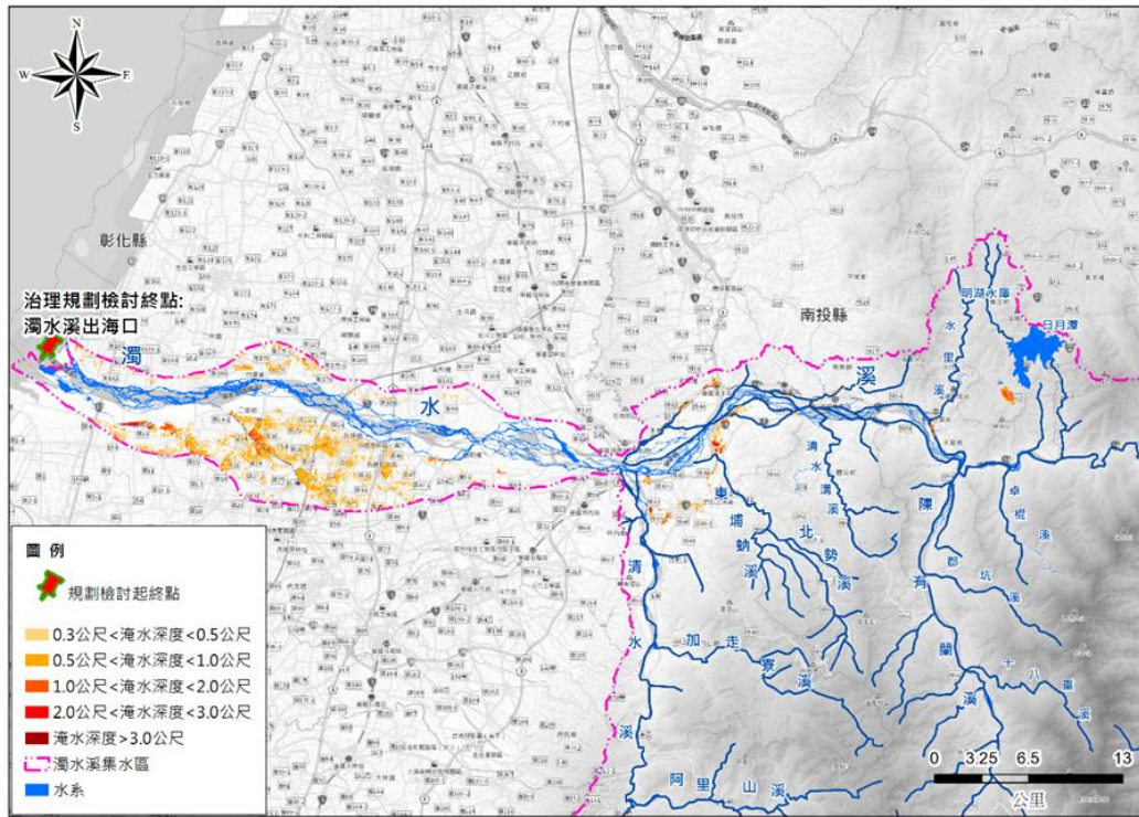
圖 2-13 濁水河流域 24 小時下降 650 毫米降雨狀況淹水潛勢圖
