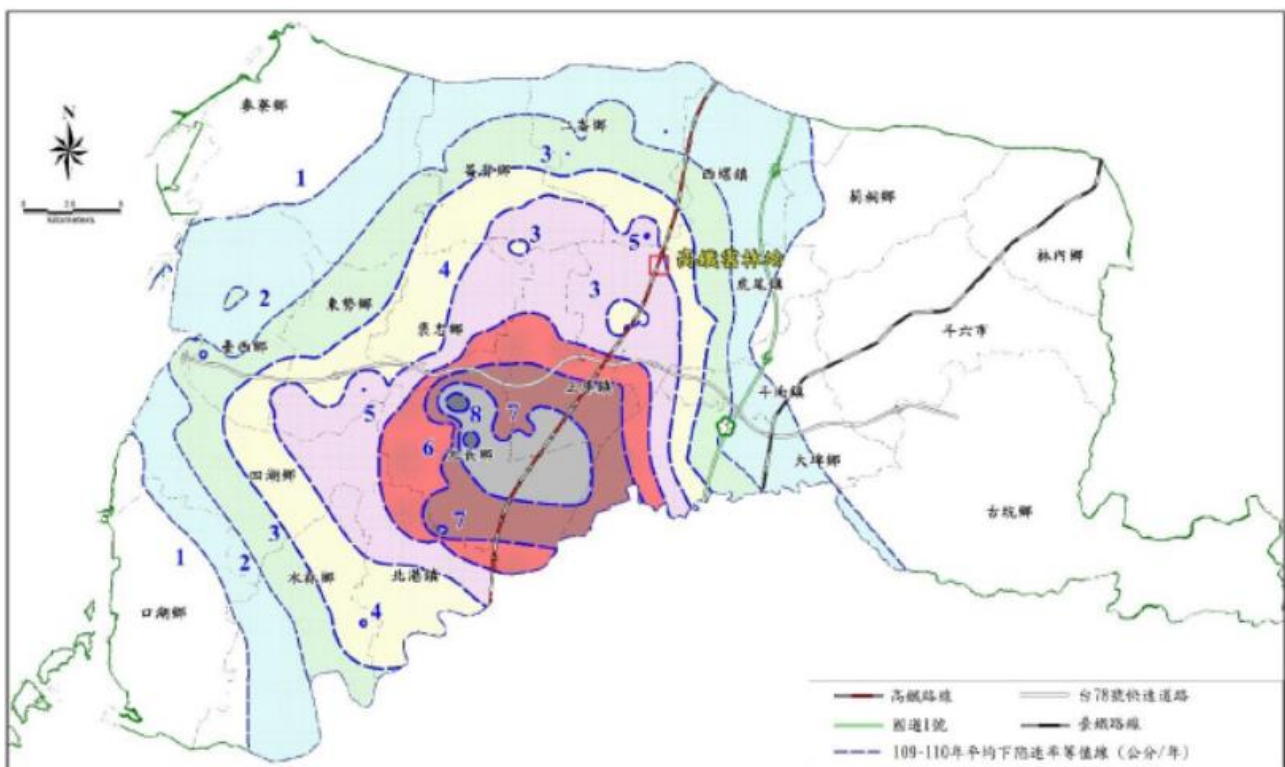
圖 2-54 雲林地區 109/4~110/9 平均下陷速率圖
