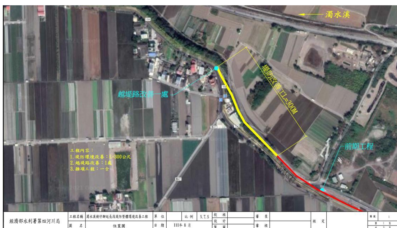
圖 2-64 樹仔腳堤防整體環境改善工程規劃圖
