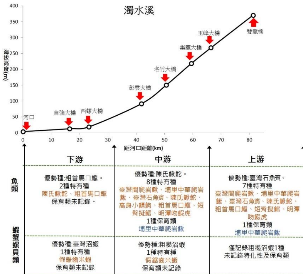
圖 2-58 濁水溪主流水域生物種類分布圖
