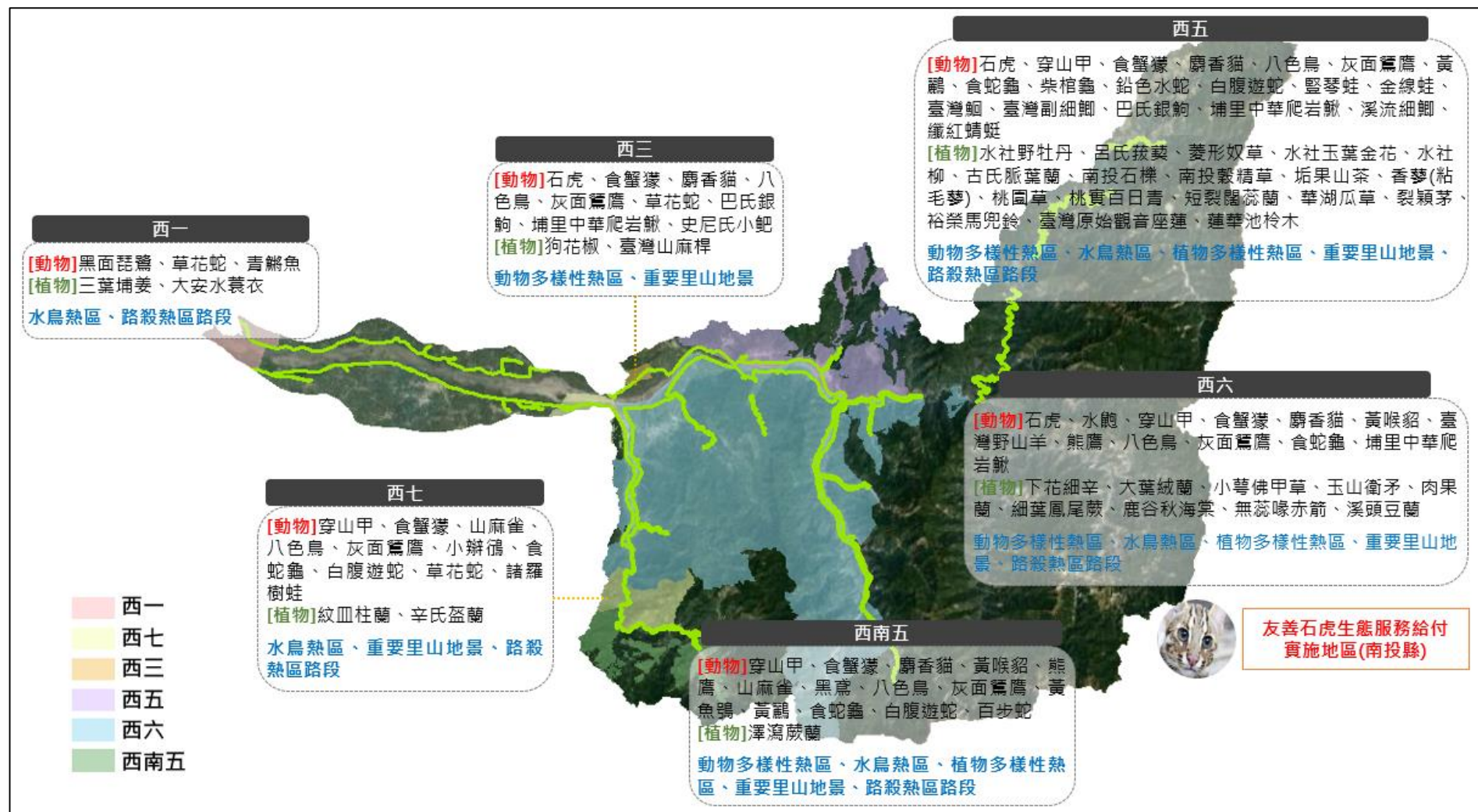
圖 2-56 濁水河流域綠網關注區域及重要關注物種分布圖
