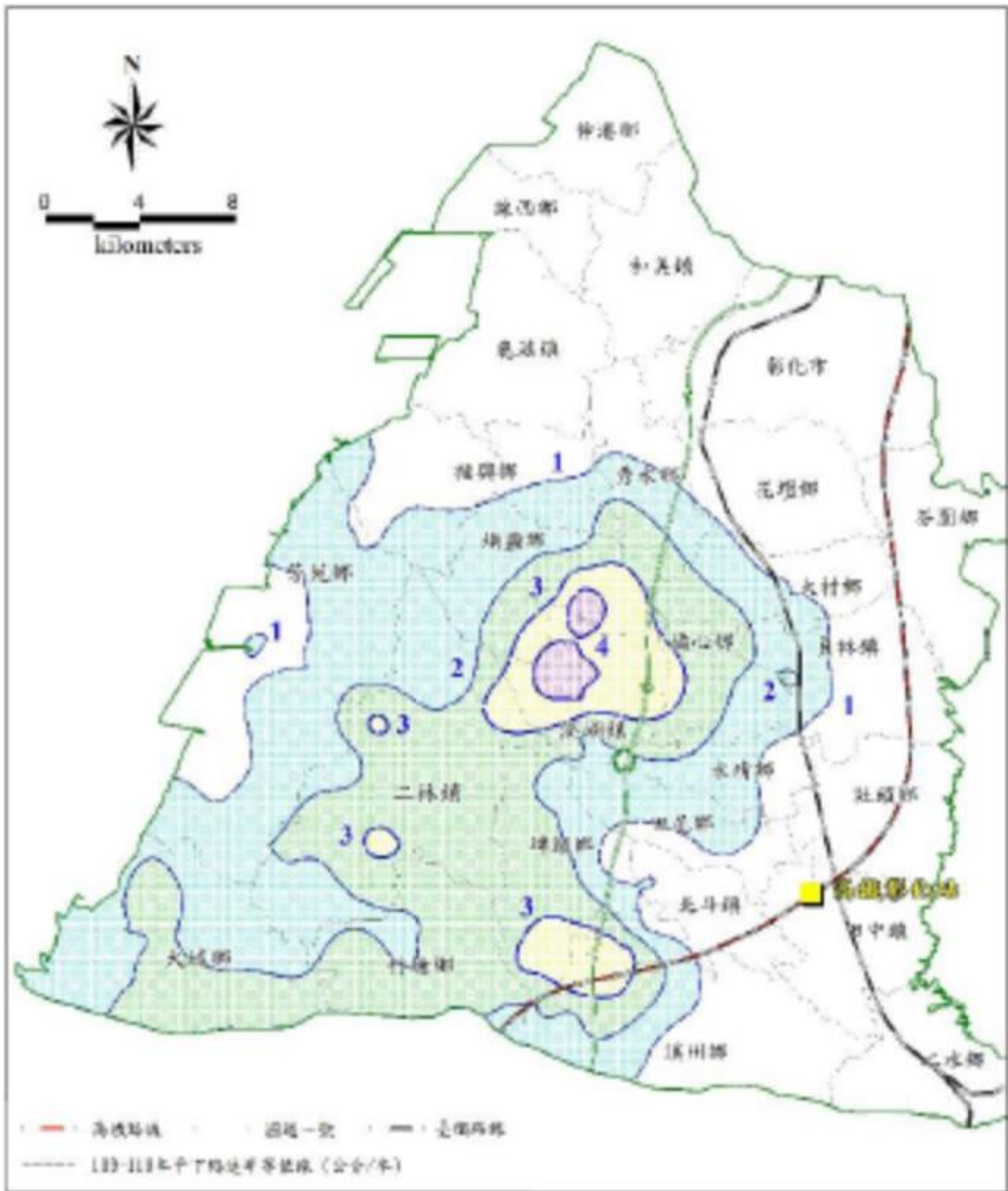
圖 2-52 彰化地區 109~110 平均下陷速率圖
