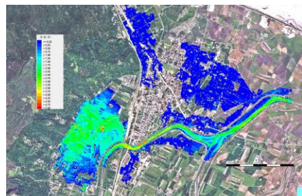
光復溪區域排水內水之淹水情況(Q100)
