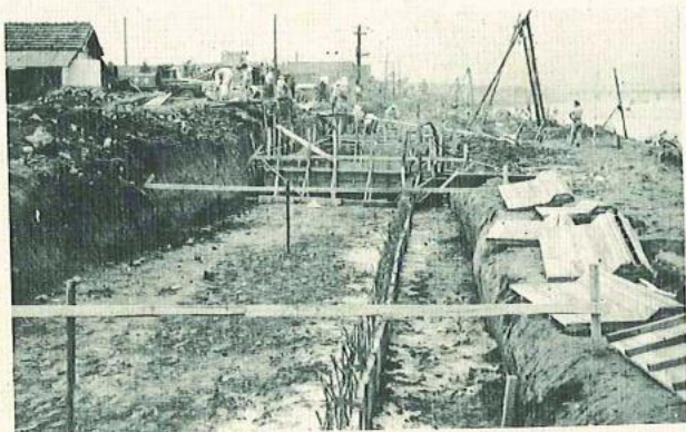
工施礎基
