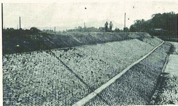
貌 全 堤 路
