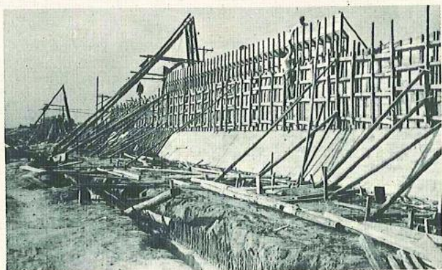
灌築防洪牆
