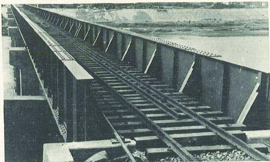
橋 路 鐵 山 圓
