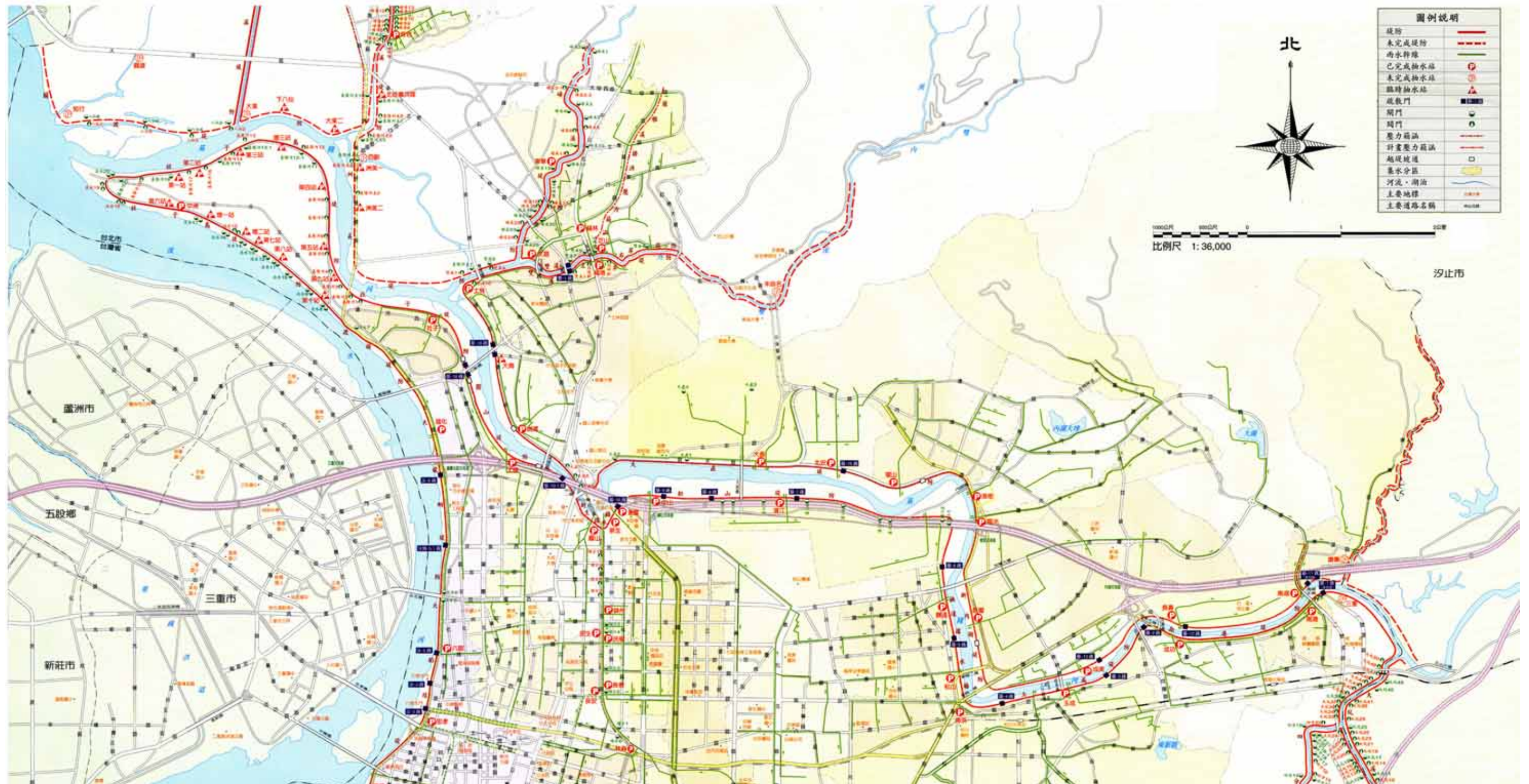
圖4-3 基隆河台北市轄區防洪設施佈置圖
