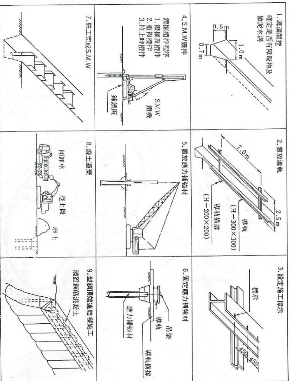
圖十二 施工程序 (以擋土牆為例)
