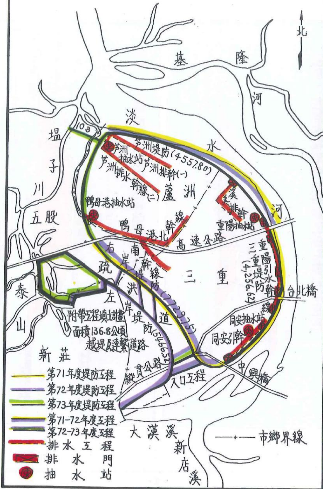
圖三 台北地區防洪計畫初期實施計畫工程佈置圖
