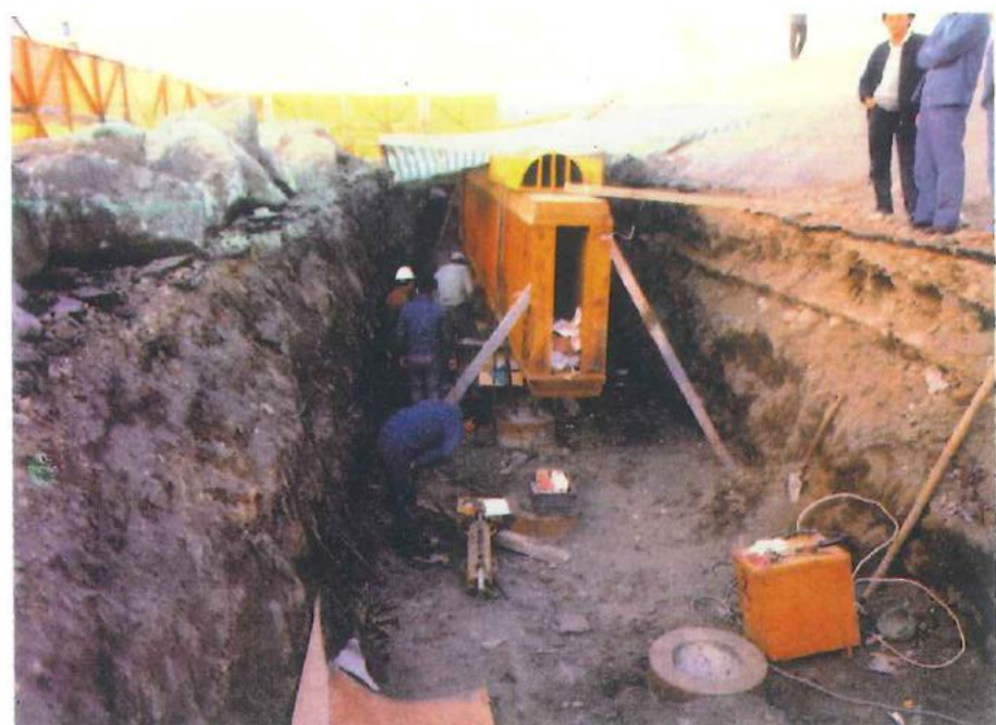
防洪牆基礎荷重試驗
