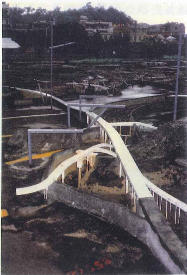
照14 溪水河水工模型基隆河中山橋河段橋墩密佈
