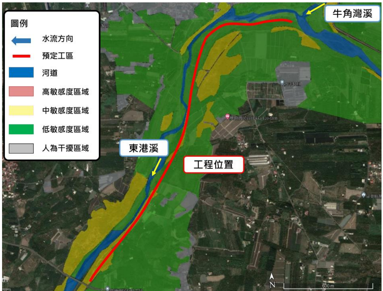
圖 2-3 東港溪成德護岸段改善工程生態關注區域圖
