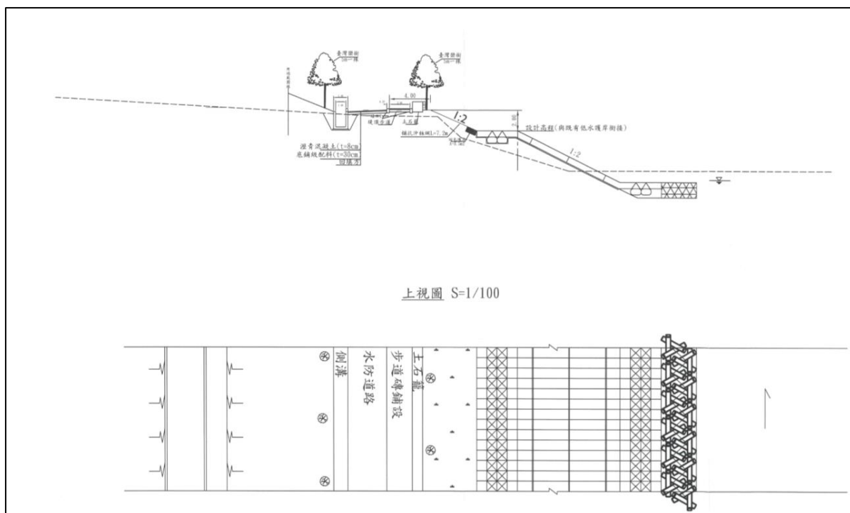
圖 1-2 東港溪成德護岸段改善工程斷面圖
