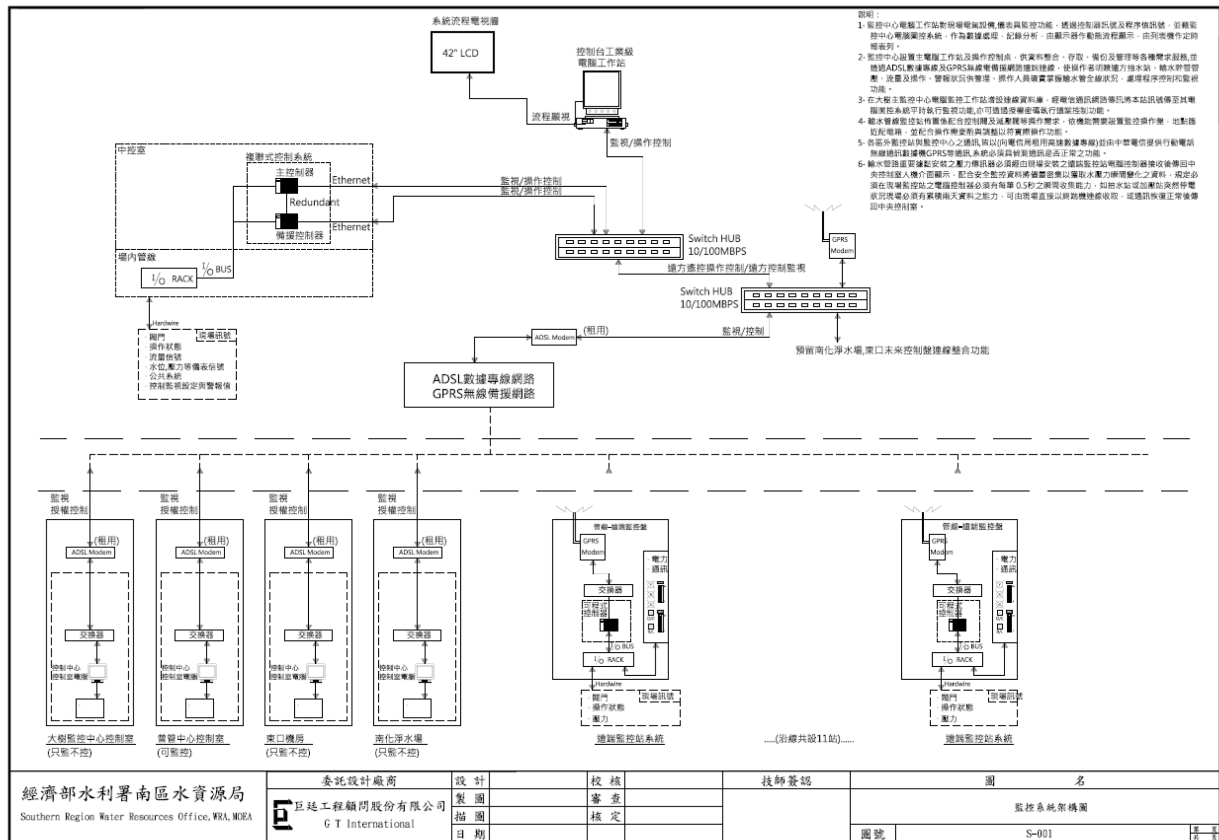
圖 6-1 本計畫監控系統架構示意圖
