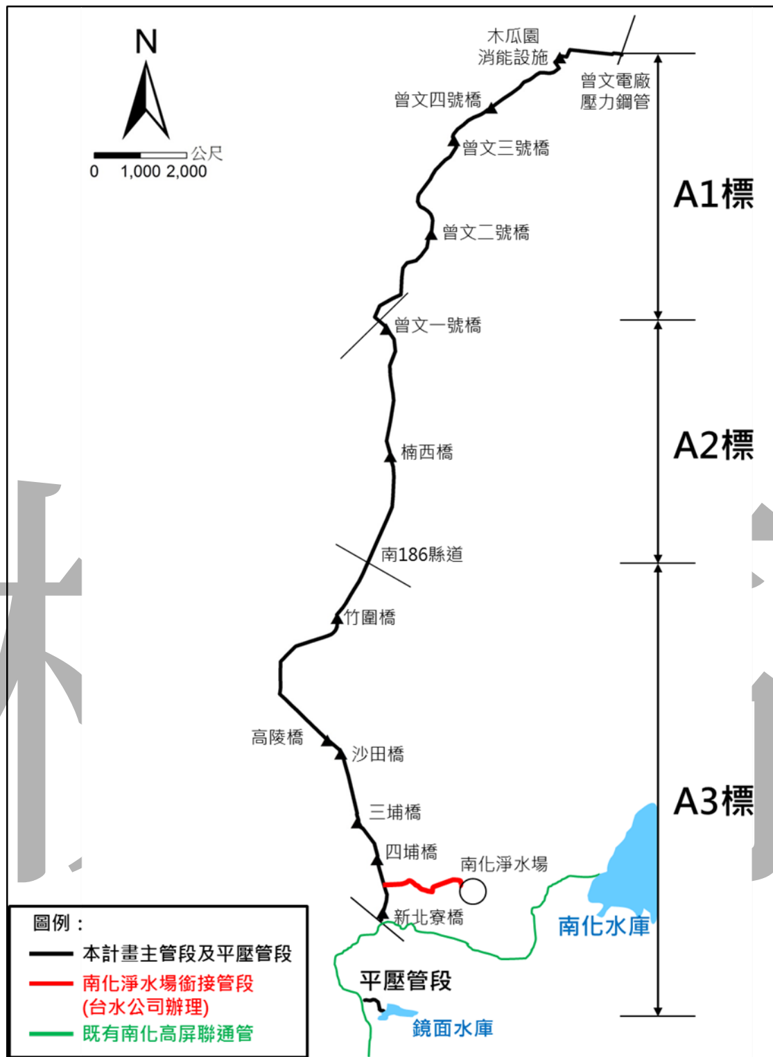
圖 1-2 工程分標示意圖
