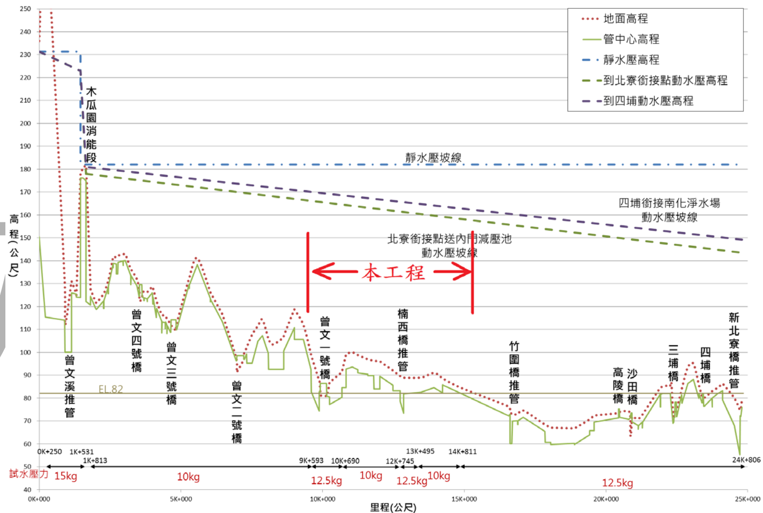
圖 3-1 曾文南化聯通管輸水 80 萬 CMD 水力坡降線示意圖
