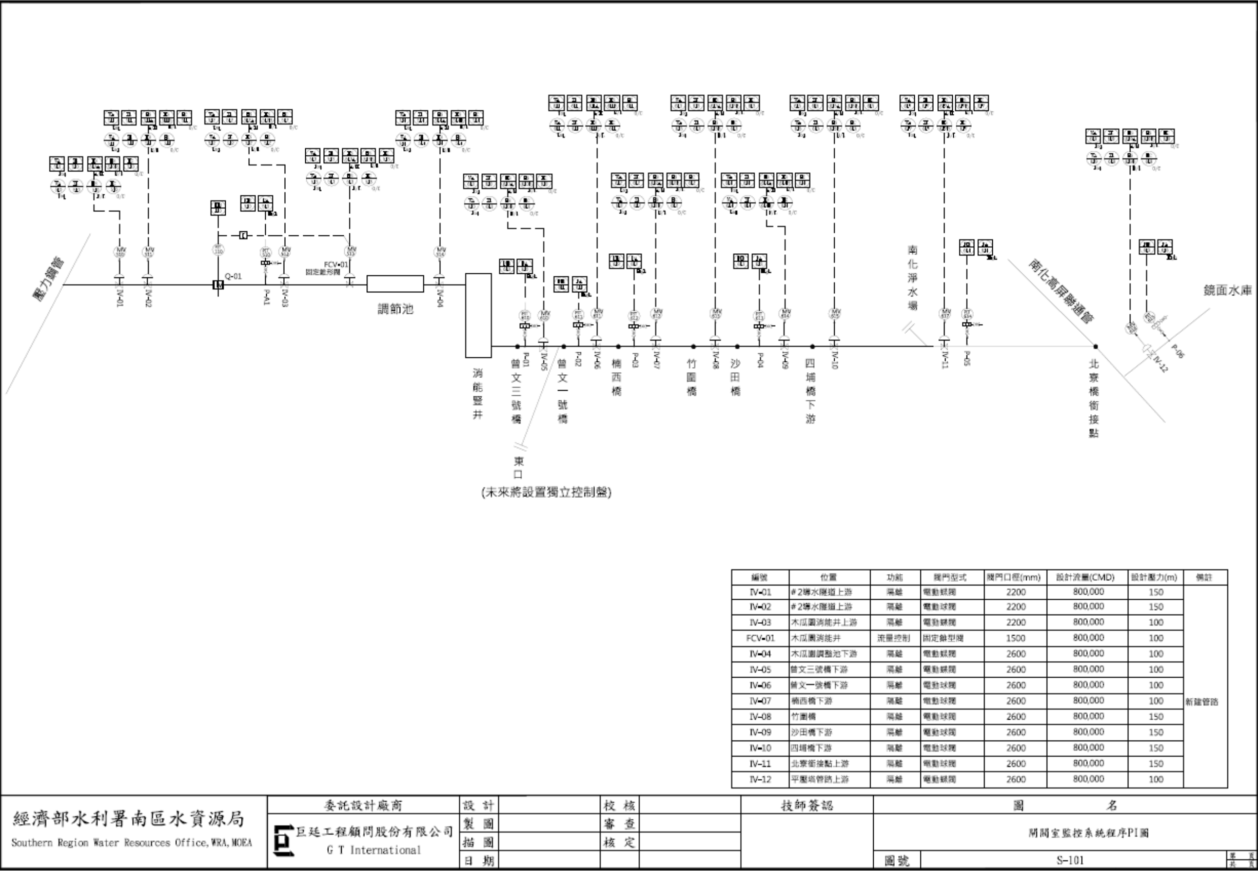
圖 6-2 本計畫監控系統程序控制 P&I 示意圖
