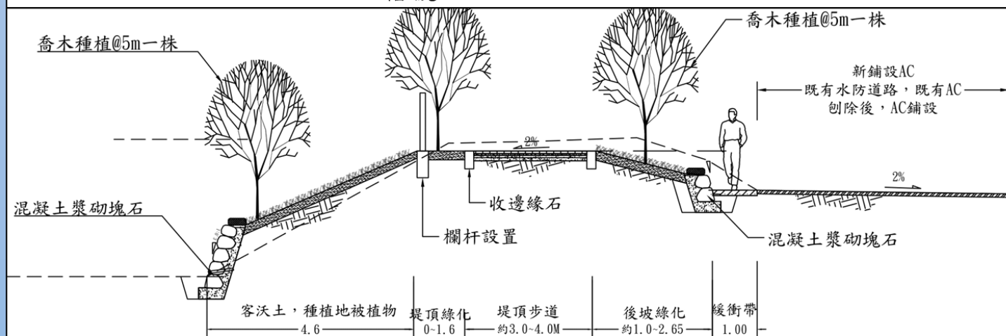
標準斷面圖(四)
