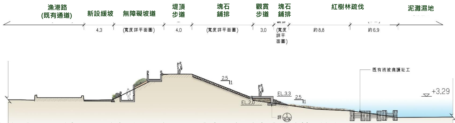
王功新生地海堤漁港段環境改善標準斷面圖
