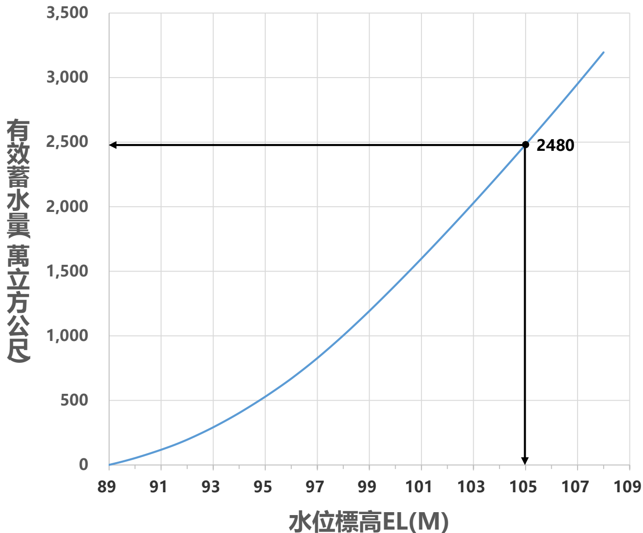
仁義潭水庫水位-蓄水量對照圖
