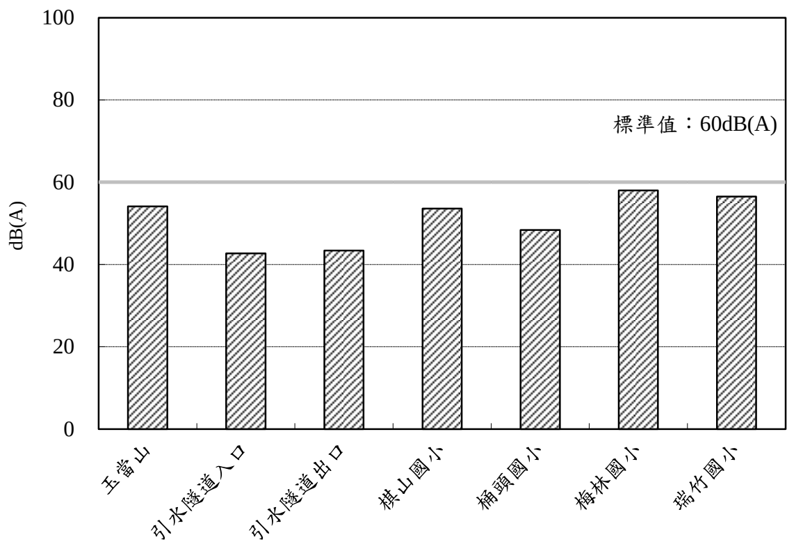
圖 2.2-1 本季噪音均能音量 L_{\text{日}} 比較圖
