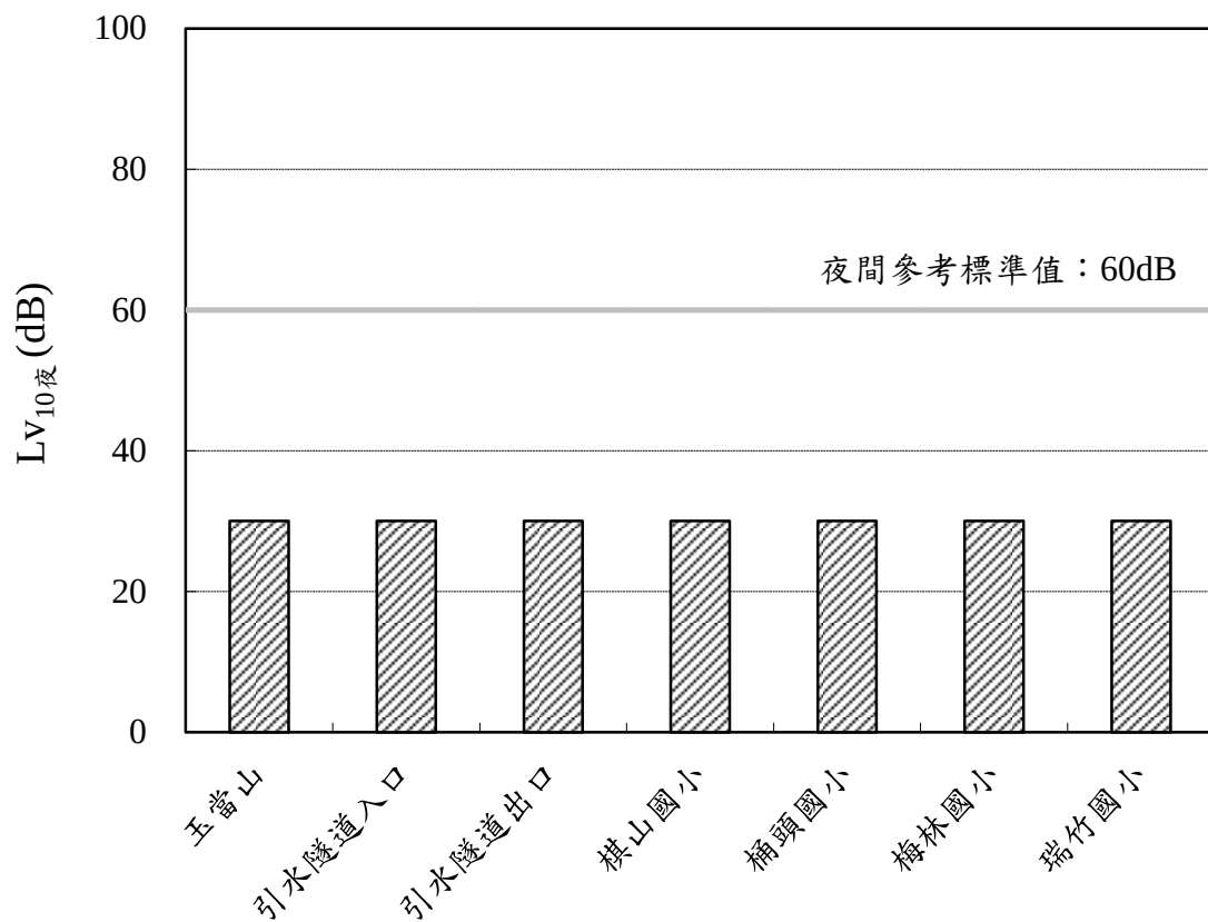
圖 2.2-5 本季夜間 L_{v10} 振動監測結果比較圖
