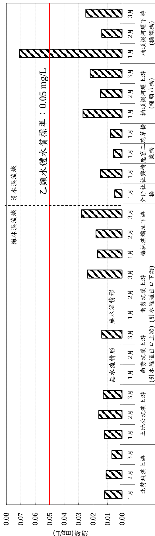
圖 2.3-6 本季河川水質懸浮固體監測結果比較圖
