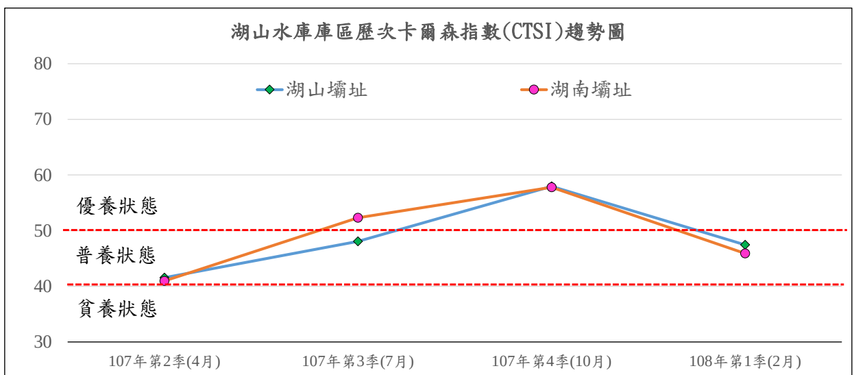
圖 3.1-6 湖山水庫庫區歷次 CTSI 變化
