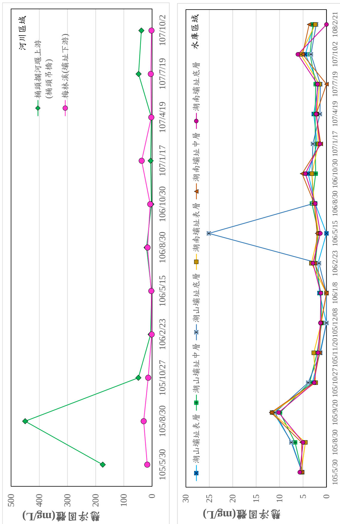
圖 2.3-40 歷次地面水質懸浮固體監測成果比較圖
