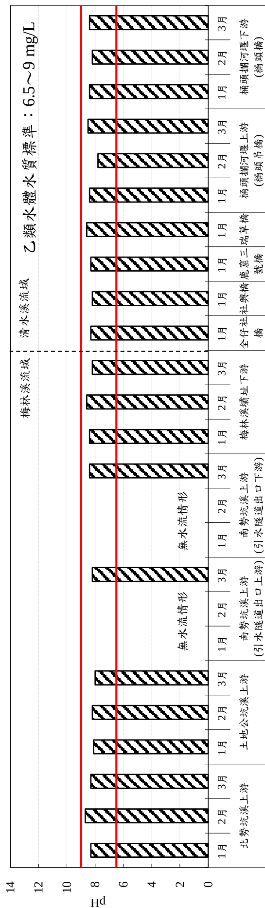
圖 2.3-2 本季河川水質 pH 監測結果比較圖
