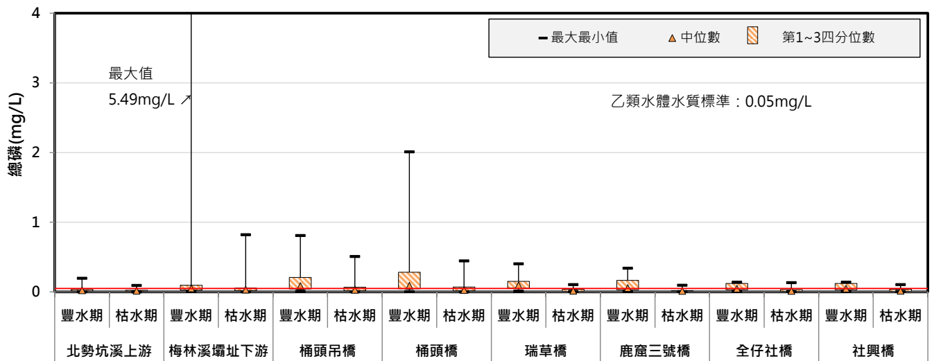
圖 3.1-4 本計畫河川水質之總磷歷年成果圖
