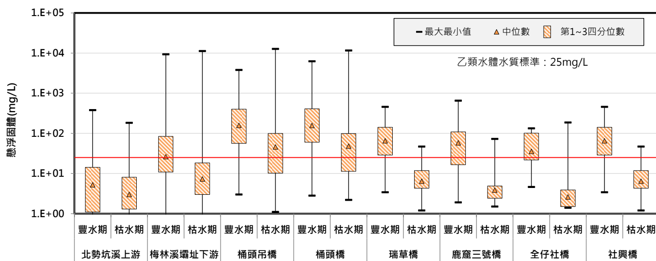
圖 3.1-1 本計畫河川水質之懸浮固體歷年成果圖
