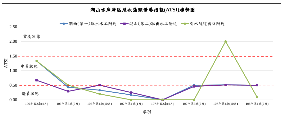
圖 3.1-7 湖山水庫庫區歷次 ATSI 變化
