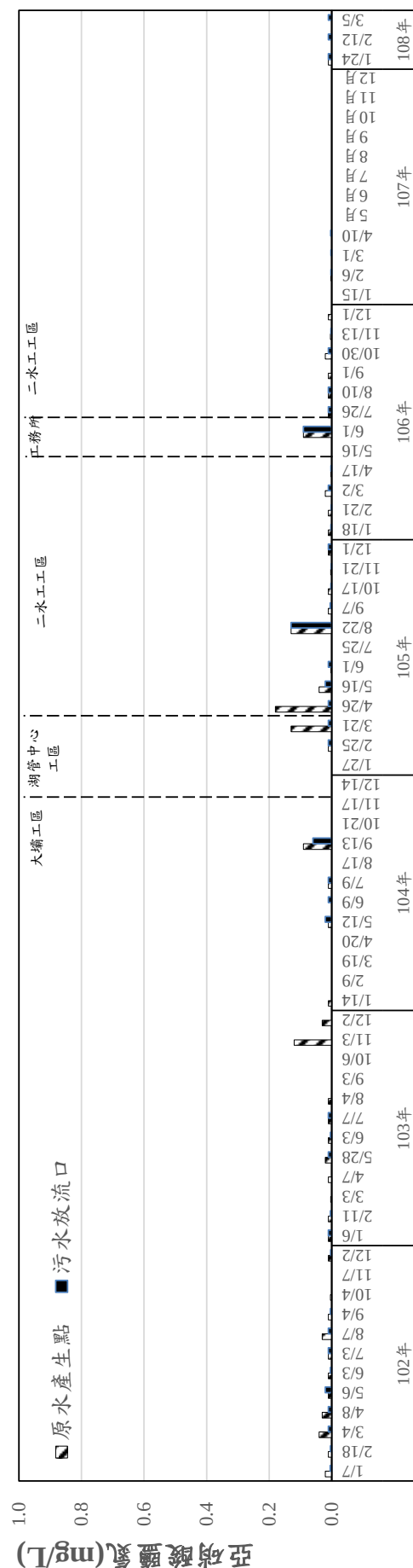
圖 2.3-27 歷次工地水質硝酸鹽氮監測結果比較圖
