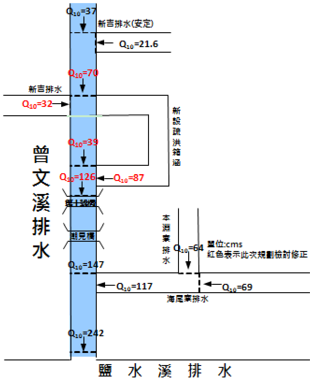
圖 5.22 本次規劃檢討計畫流量分配圖
