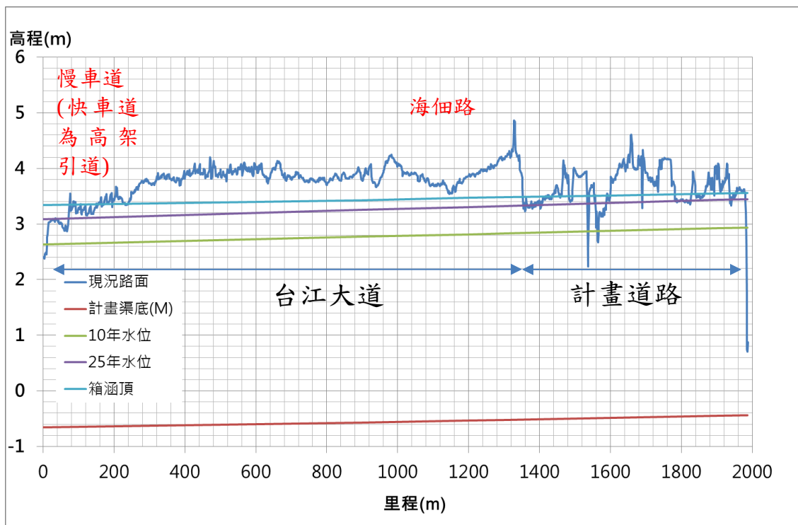
圖 5.20 曾文溪排水新設箱涵與路面高程關係圖
