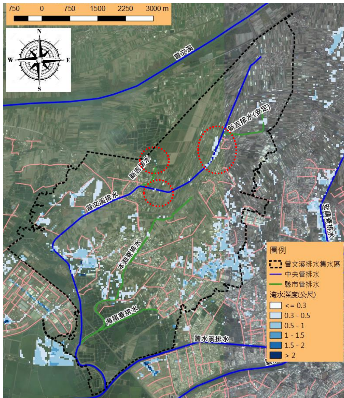
改善前 10 重現期距最大淹水範圍圖
