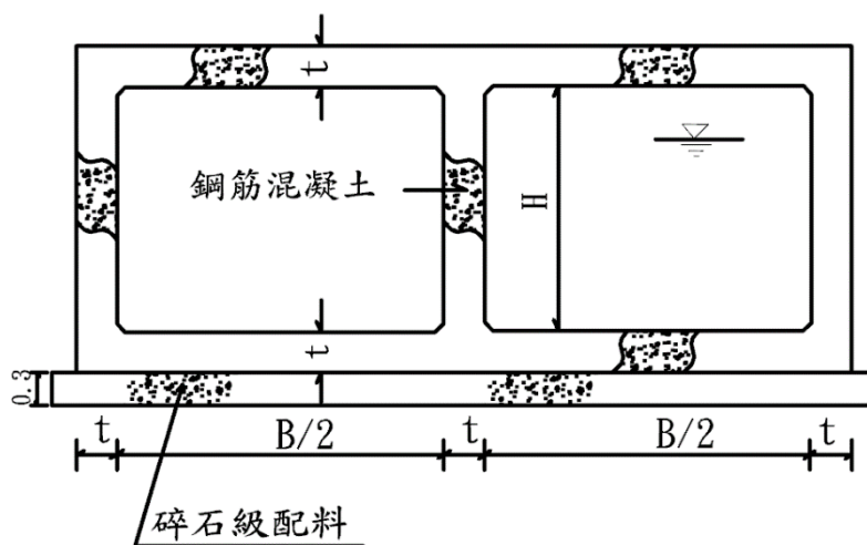
圖 6.2 曾文溪排水改善參考斷面圖(雙孔箱涵)
