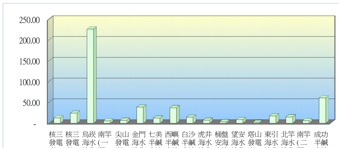
圖5 海水淡化廠實際造水量 民國93年
