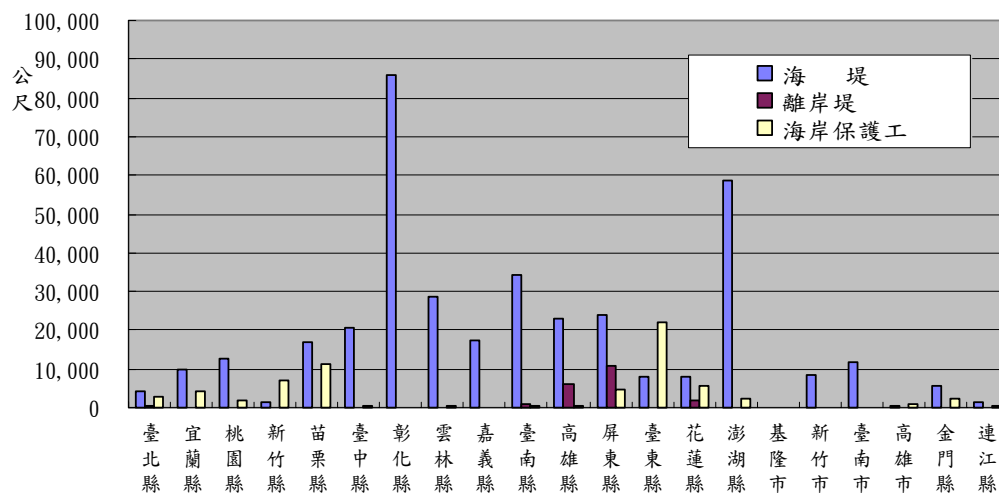
圖10 現有禦潮(海堤)設施—海堤、海岸保護工
