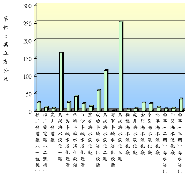
圖7 海水淡化廠實際造水量
