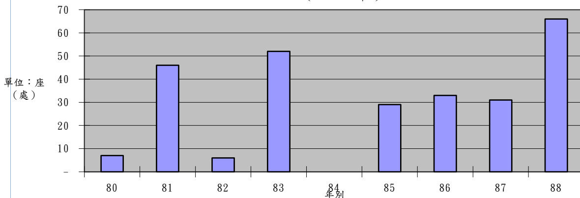
丁壩(制水門)損毀概況圖 (80-88年)
