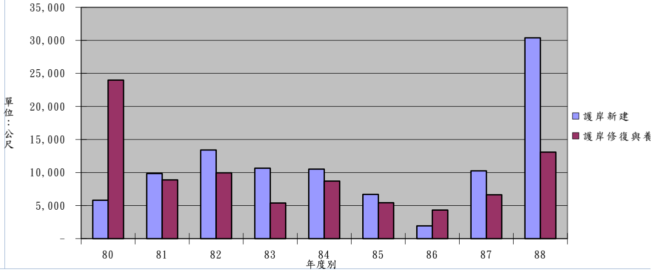
護岸損毀概況圖 (80-88年)
