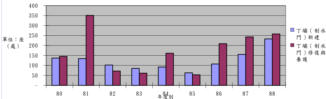
丁壩(制水門)新建、修復與養護工程概況圖 (80-88年)
