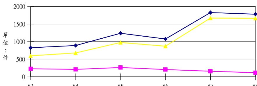
施工中工程混凝土鑽心取樣抽驗結果 -- 件數統計圖
