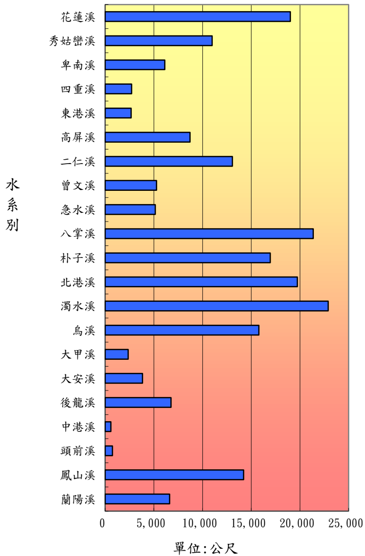
中央管河川堤防、護岸工程辦理概況-依水系別分 九十一年度
