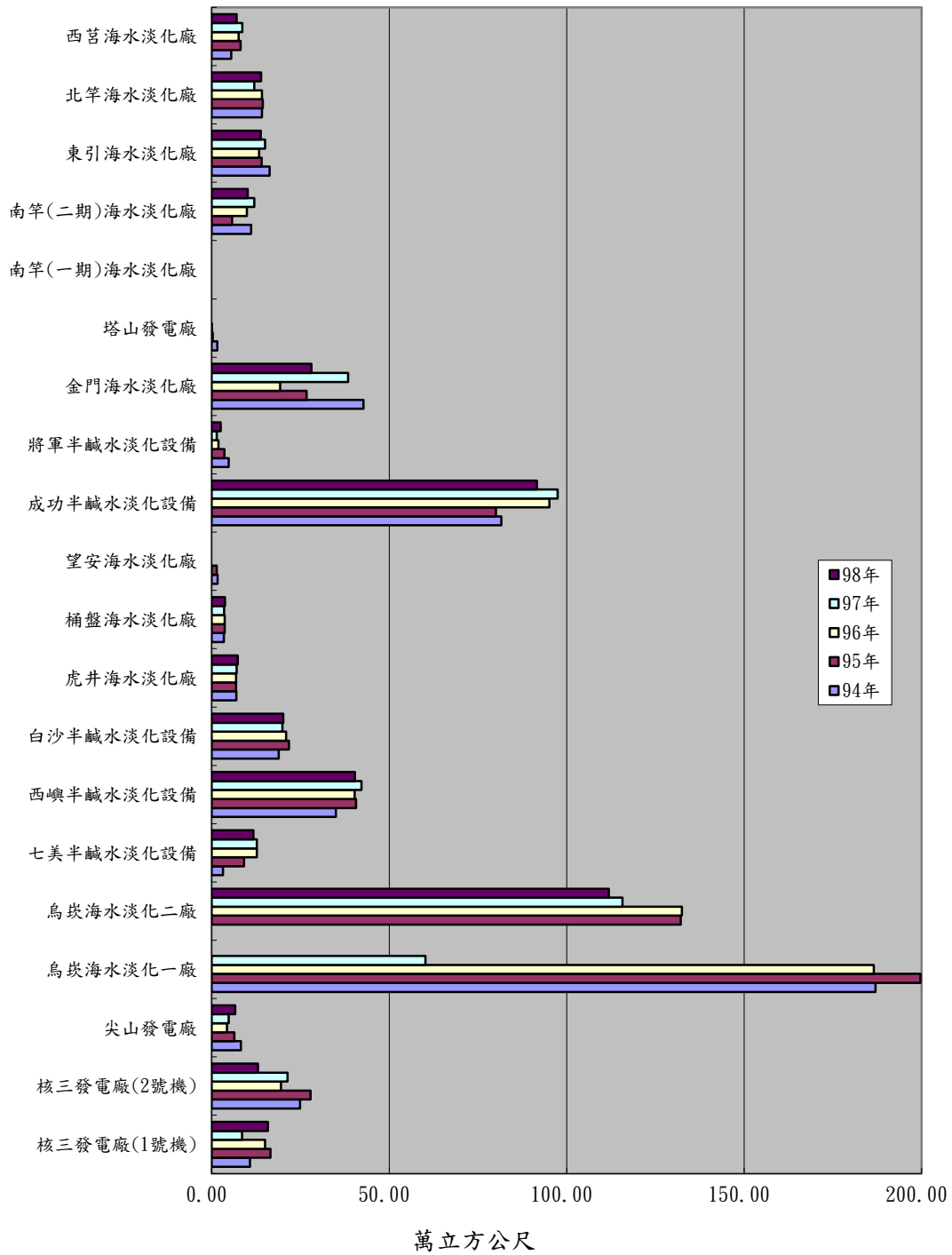
近5年海水淡化廠營運比較圖
