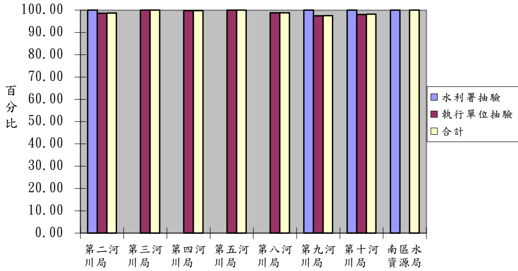
98 年施工中混凝土鑽心取樣抽驗結果統計圖
