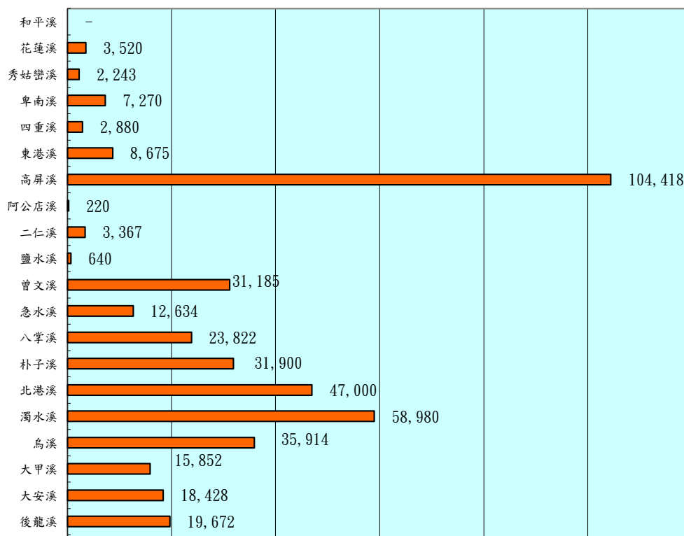
近10年中央管河川堤防、護岸損毀情形—水系別
