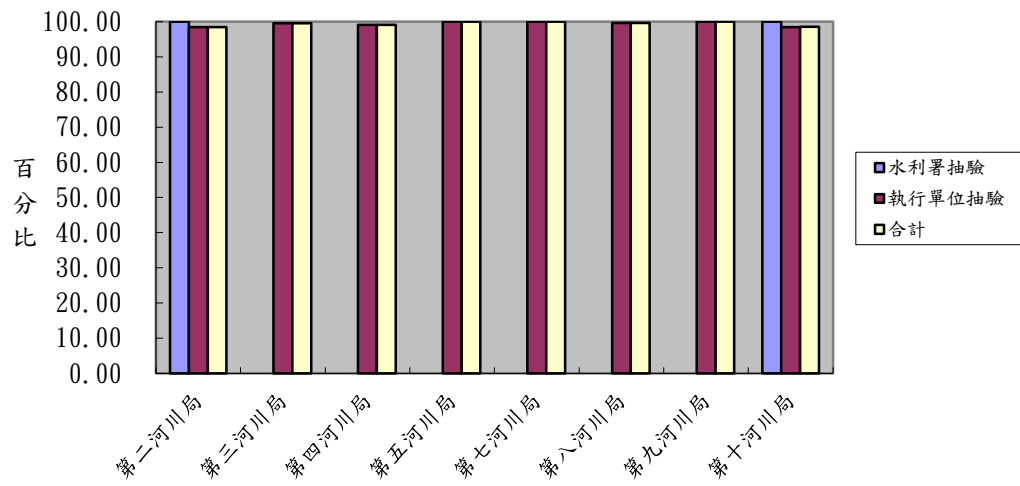
100年施工中混凝土鑽心取樣抽驗結果統計圖
