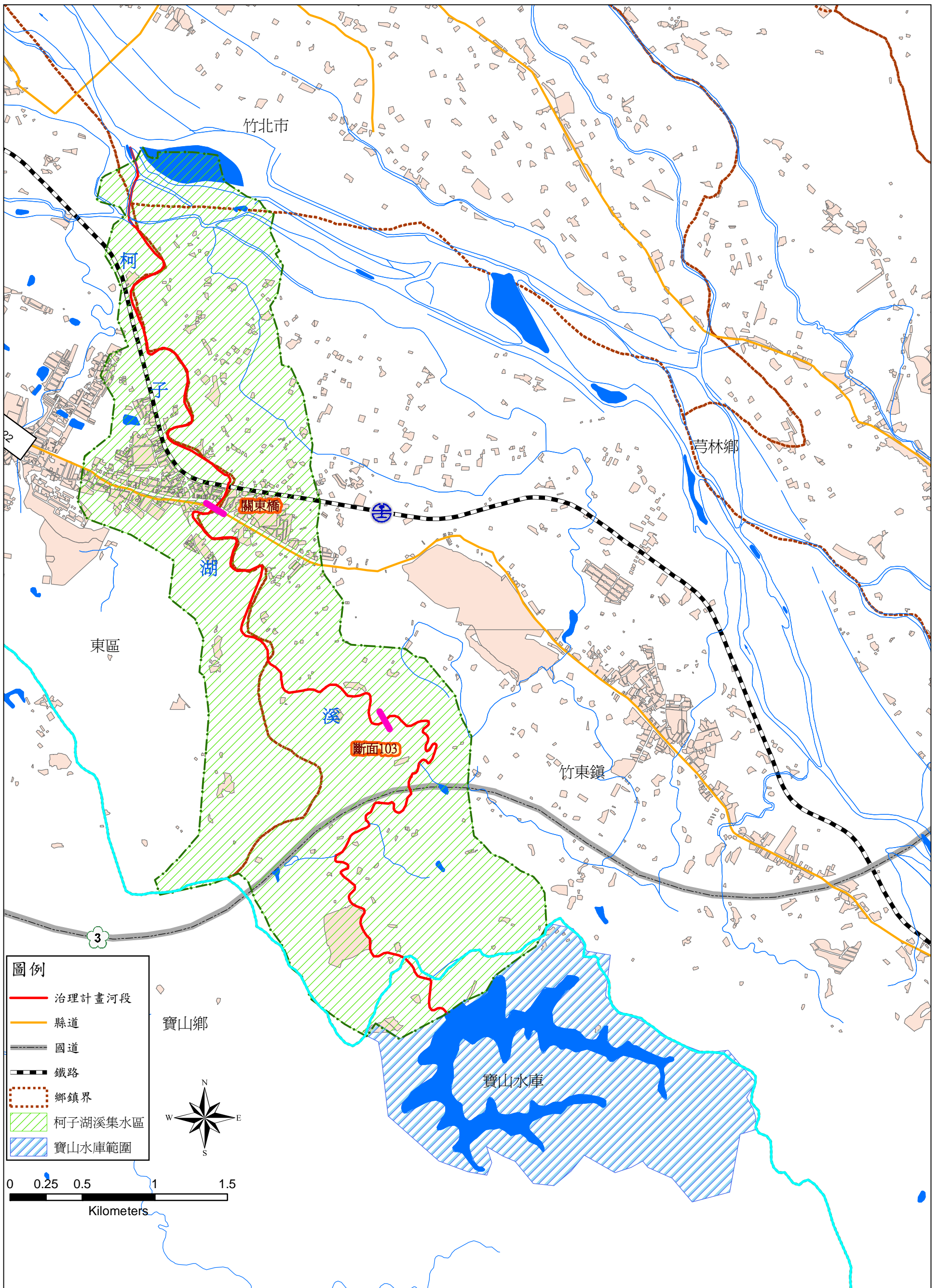
附錄一 柯子湖溪排水集水區位置圖
