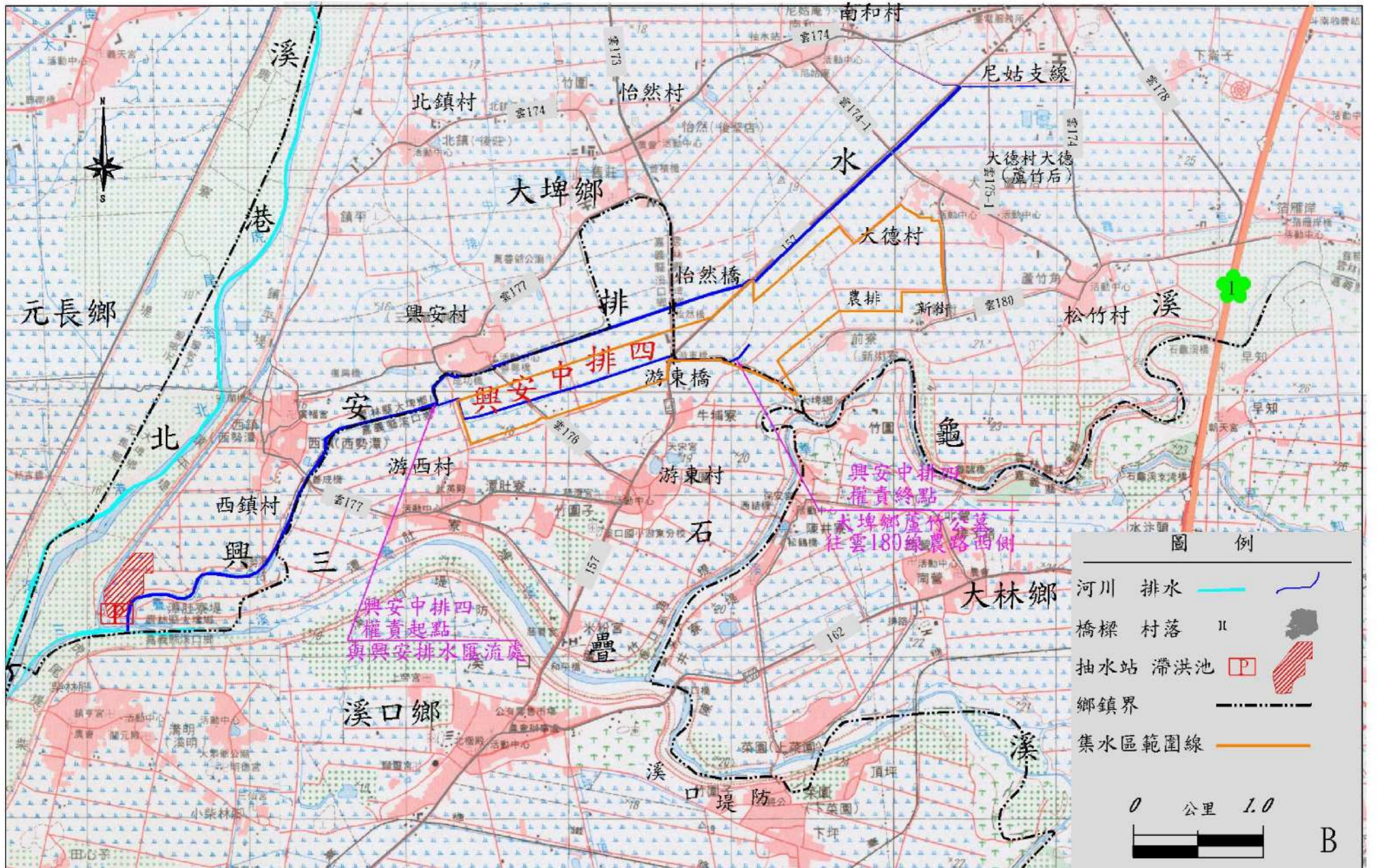
附件二 興安中排四集水區域範圍圖
