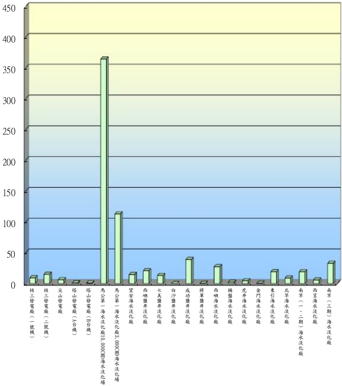
圖5 海水淡化廠實際造水量
