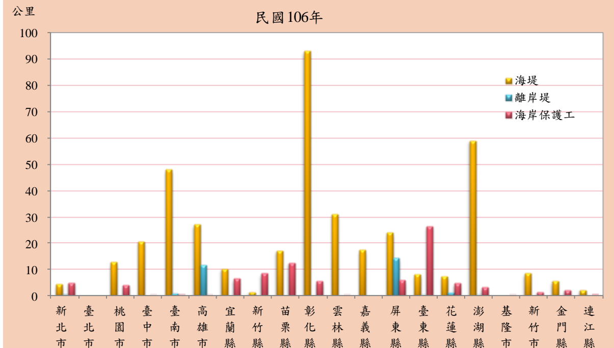
圖13 現有禦潮(海堤)設施—海堤、離岸堤、海岸保護工
