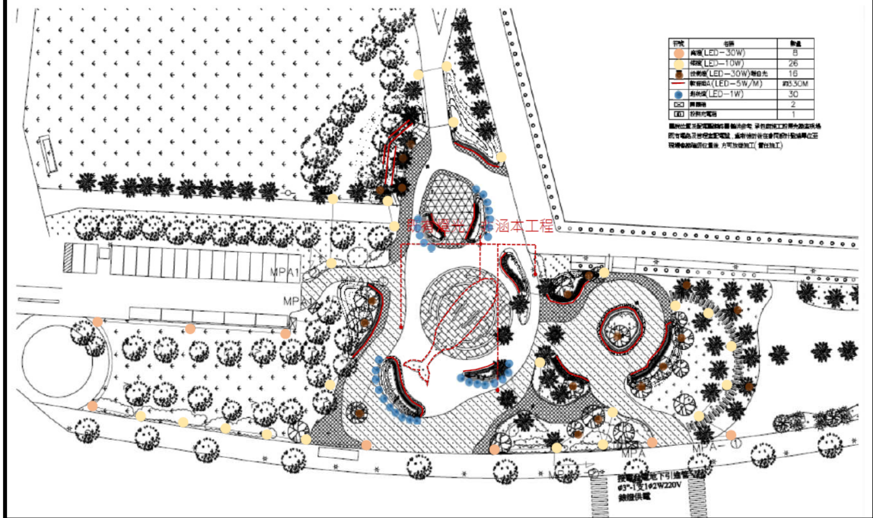
照明解說-大魚廣場照明配置圖
