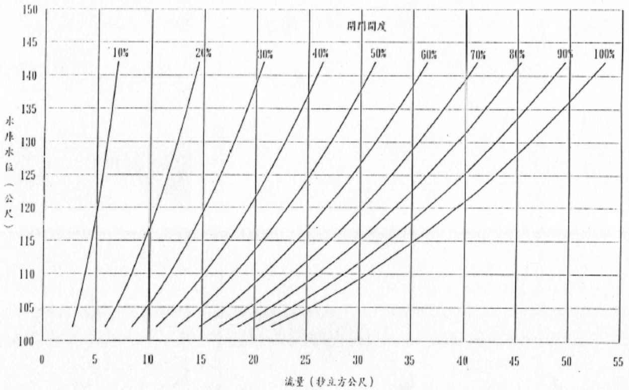
圖三：排水道控制開門開度與放流量關係曲線
