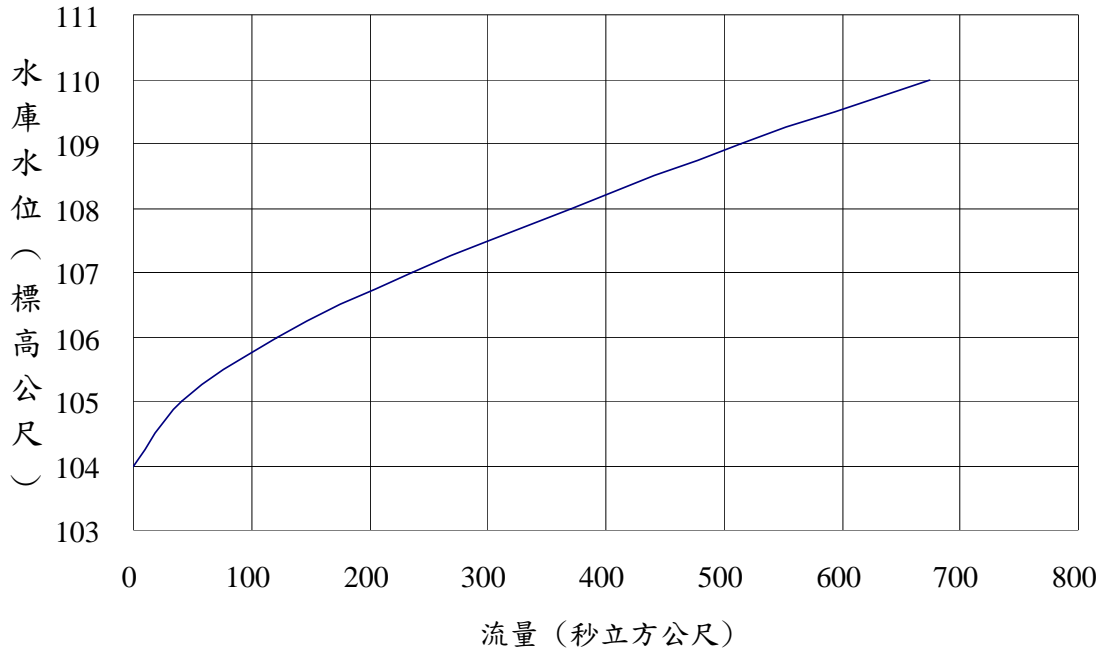
閘門全開率定曲線
