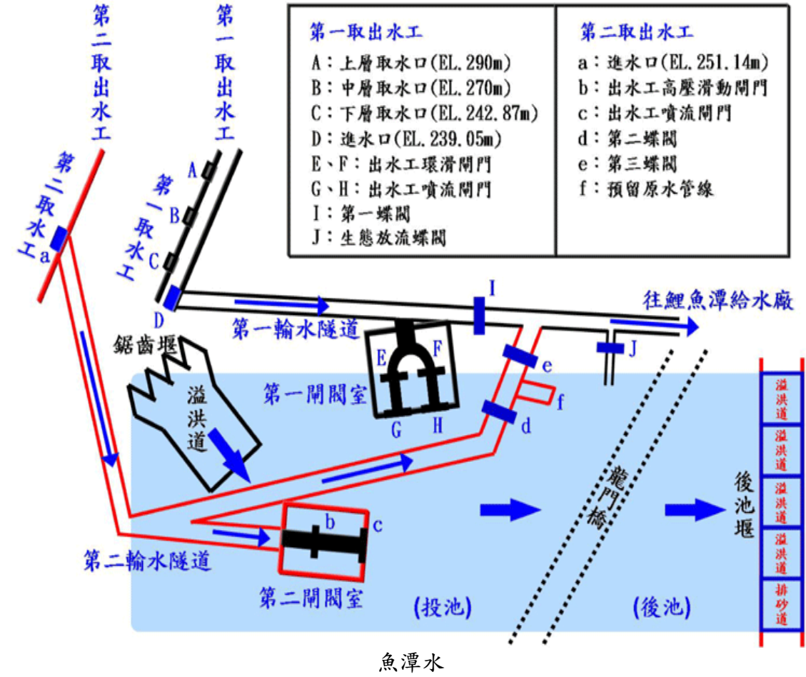
附圖、鯉庫主要設施圖
