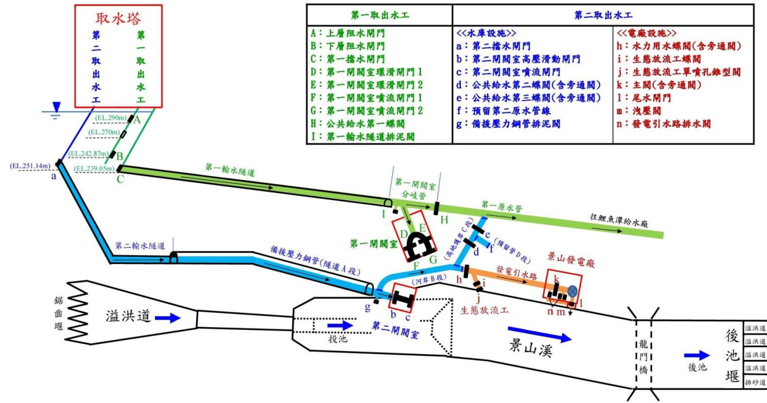
附圖、鯉魚潭水庫主要設施圖
