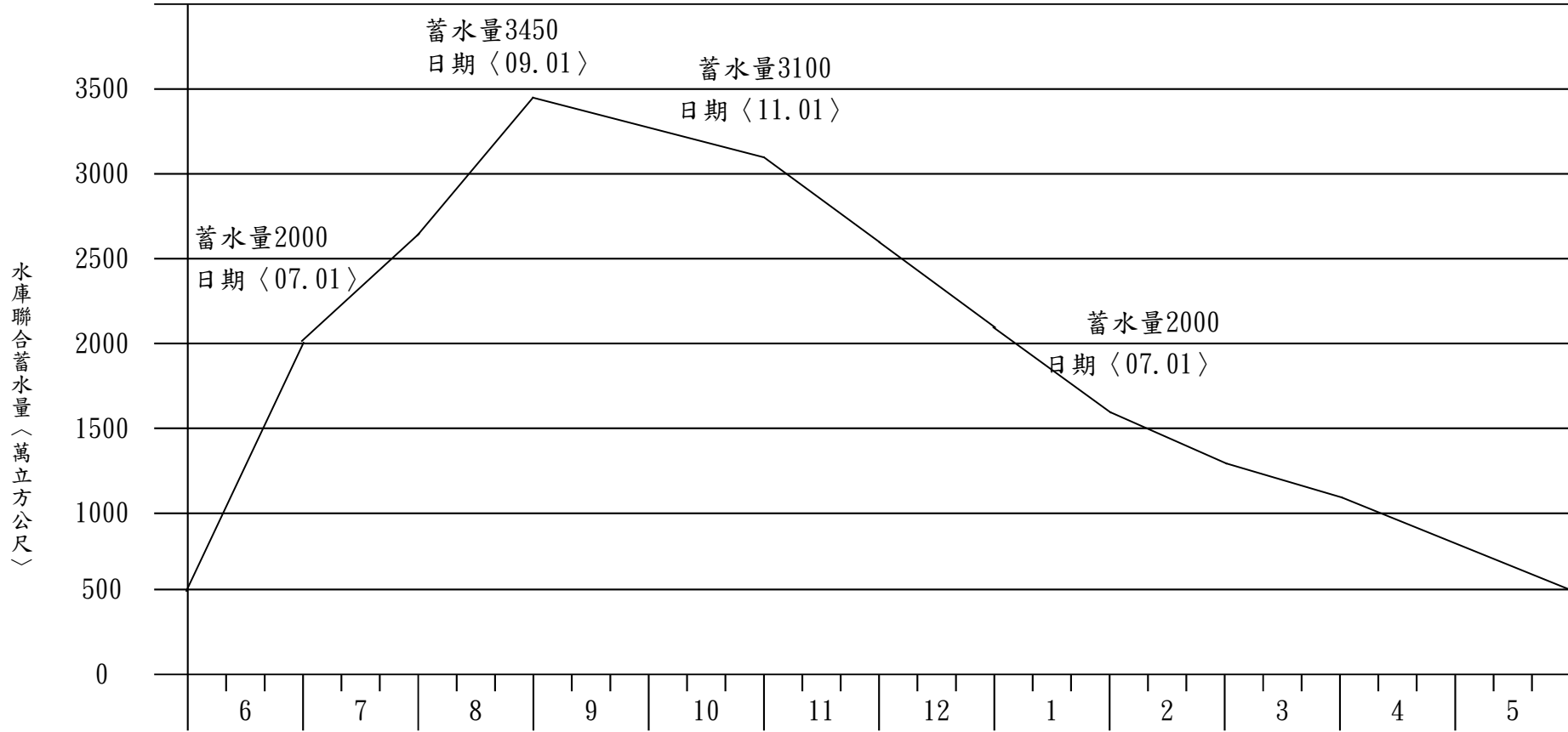
仁義潭、蘭潭水庫串聯聯合運用規線
