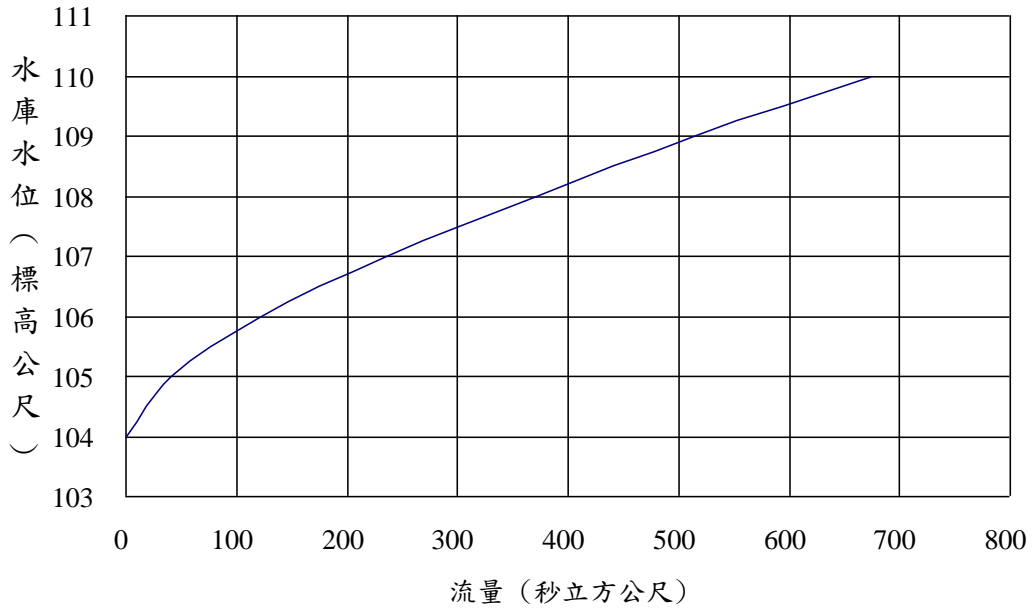
閘門全開率定曲線
