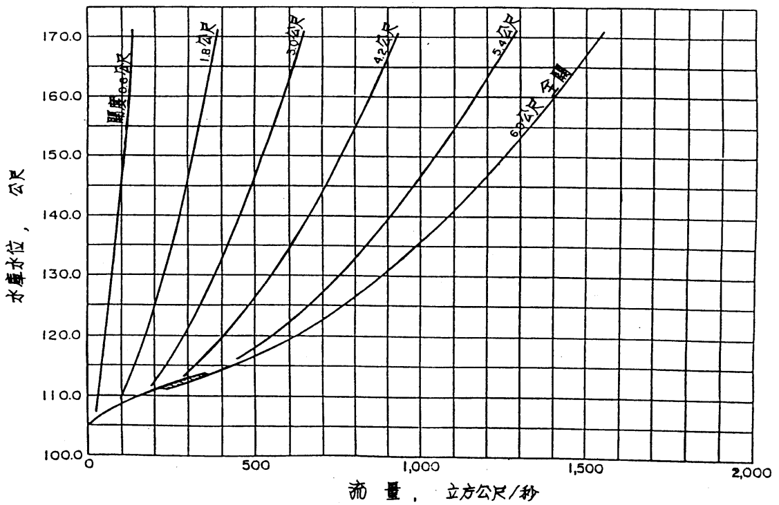
附圖三、排洪隧道閘門開度與流量關係曲線
