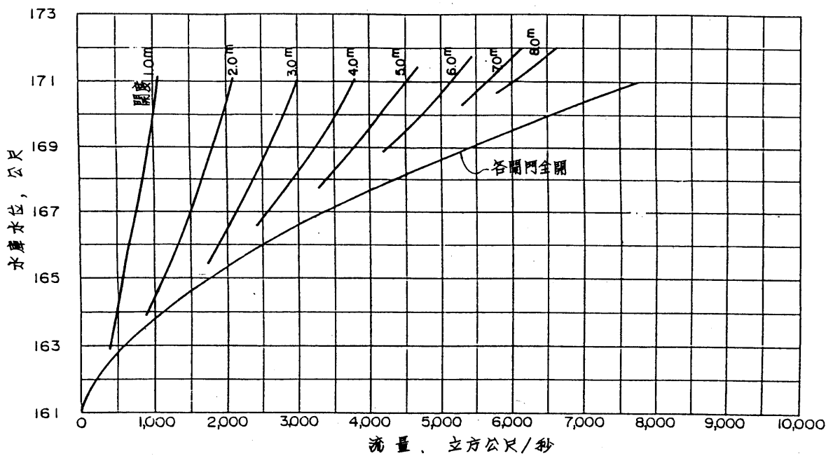
附圖一、溢洪道閘門開度與流量關係曲線
